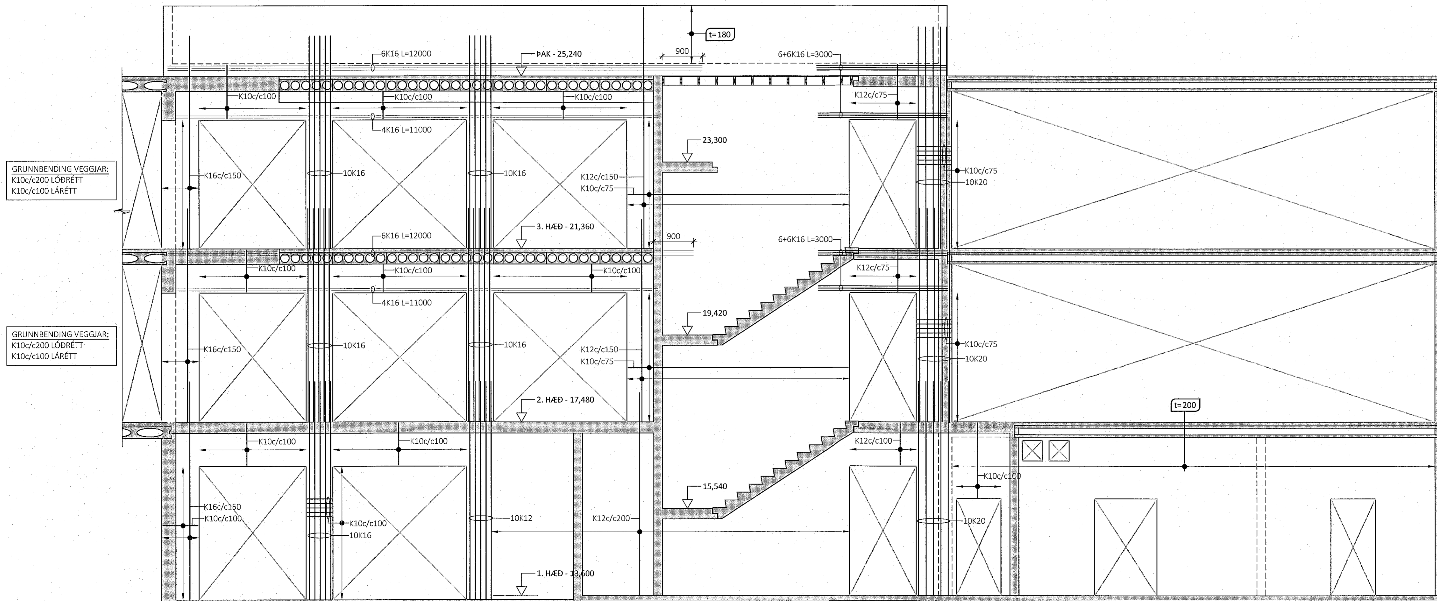
HLIDARMYND VEGGIAR V108 - M1:50: PYKKT VEGGIAR: 300mm NEMA ANNAD SÉ SÉRSTAKLEGA TEKID FRAM
