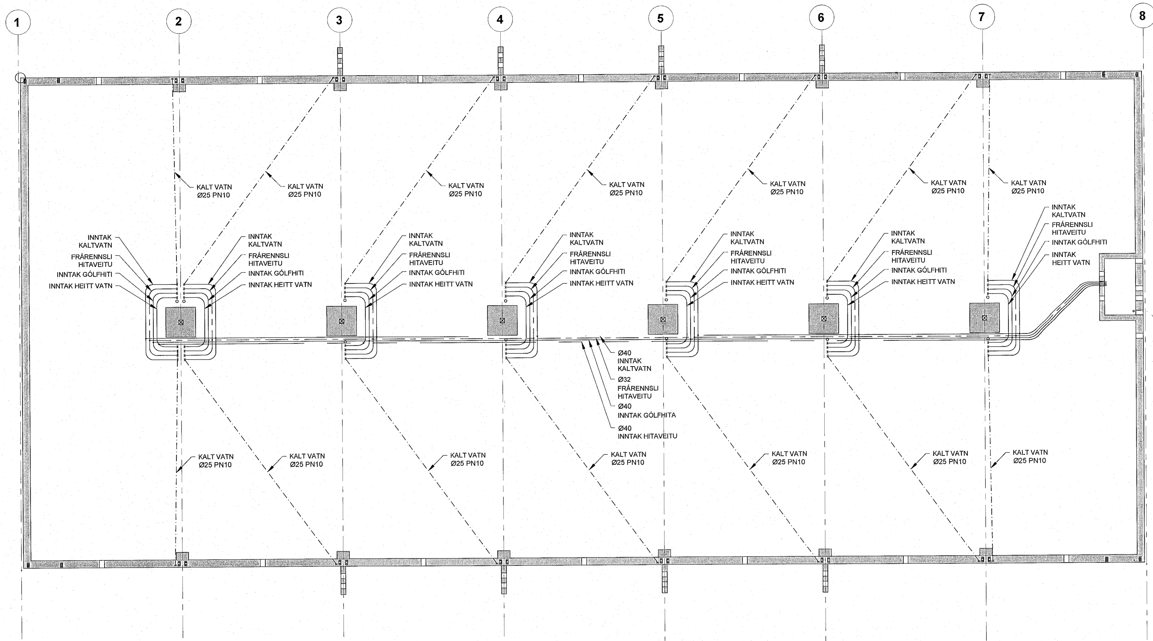
GRUNNMYND - NEYSLUVATNSLAGNIR 1:75 (A1)
