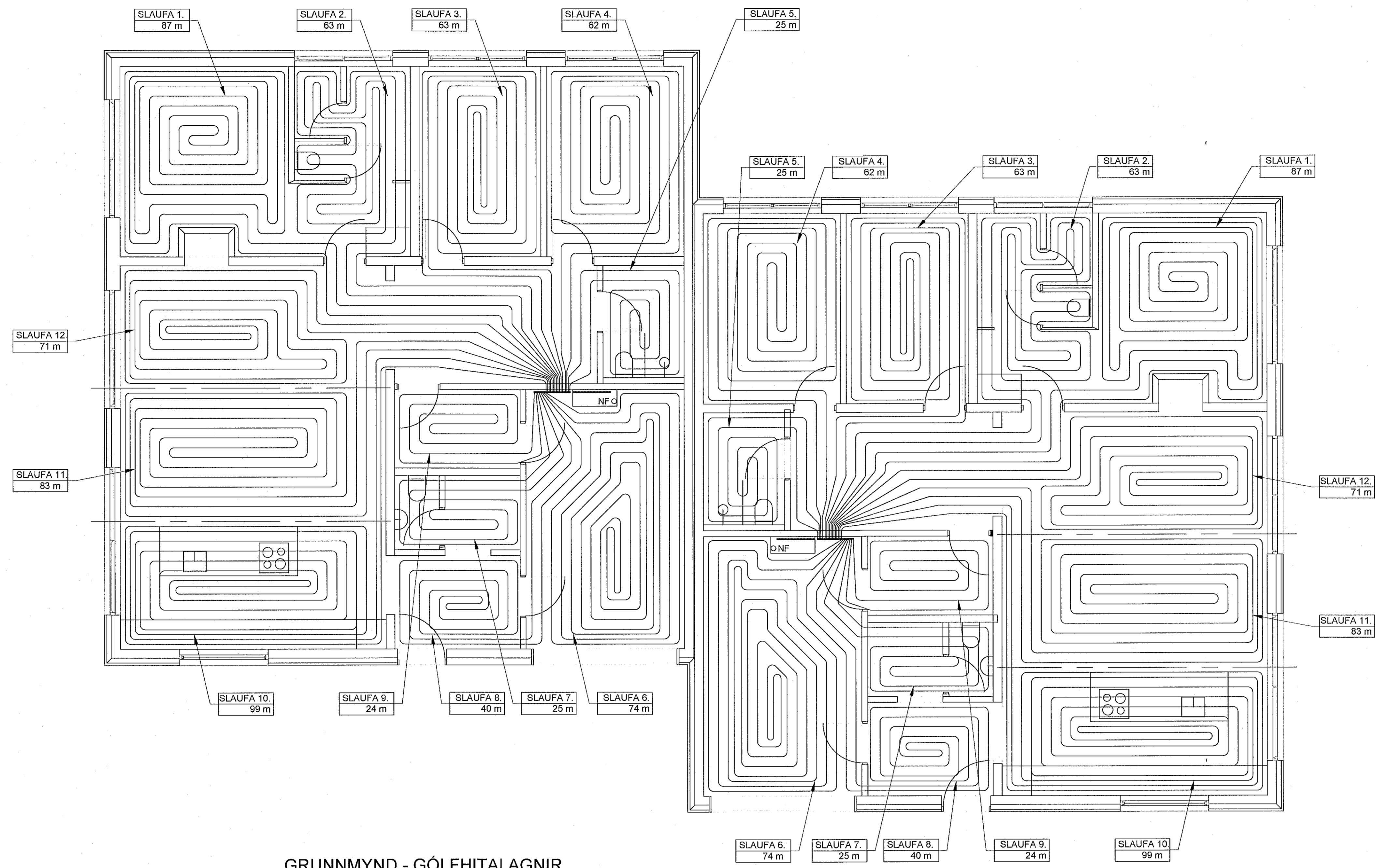
GRUNNMYND - GÓLFHITALAGNIR 1:50 (A1)
