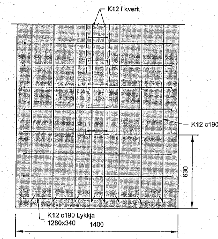
US10.1 Undirstaða 1:20
