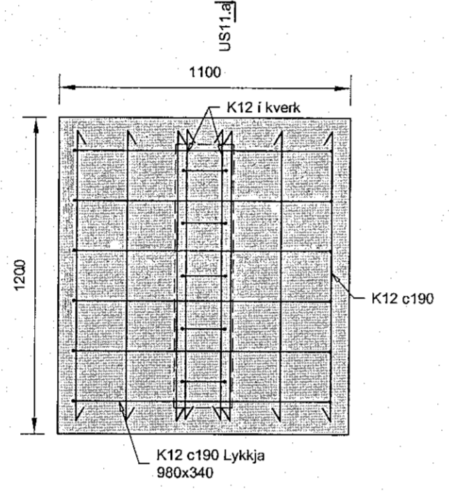
US11.1 Undirstaða 1:20
