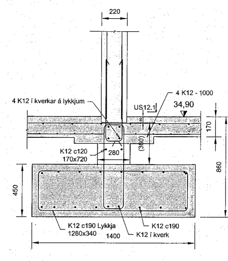
US12 Snið 1:10
