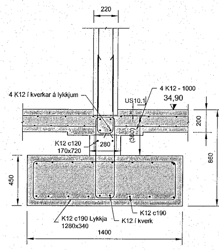
US10 Snið 1:10
