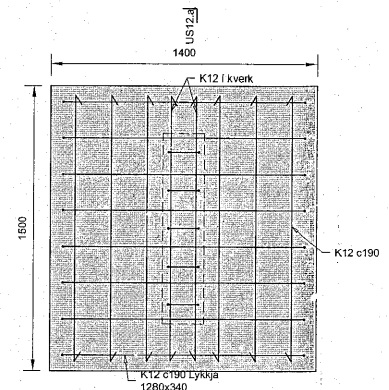
US12.1 Snið 1:20
