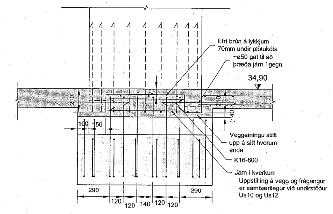
US11a Snið, uppstilling á veggveingju 1:20
