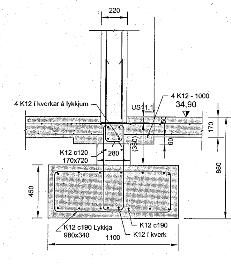
US11 Snið 1:10
