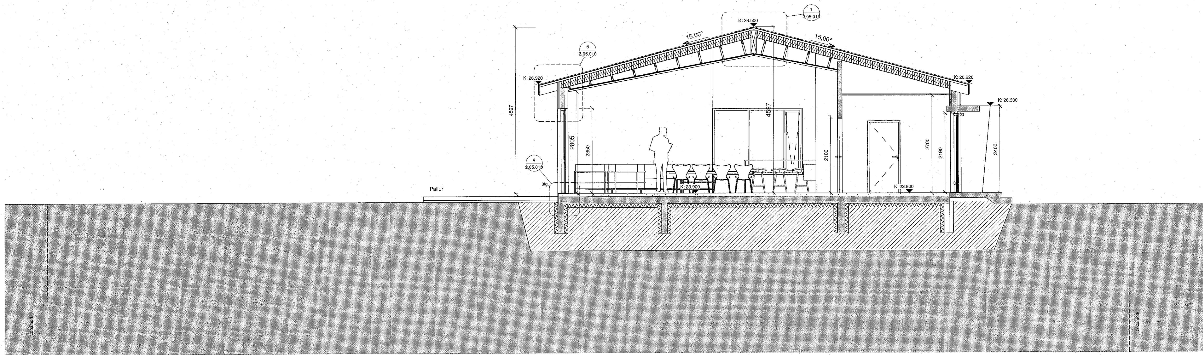
1 Sneiðmynd A Verkeikning 1:50
