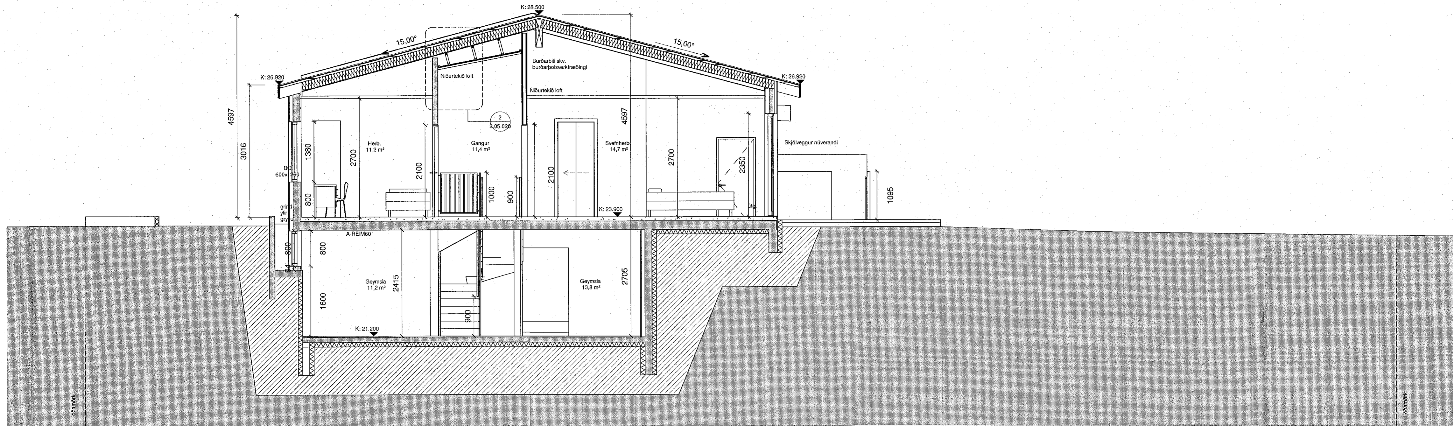
1 Sneiðmynd C Verkeikning 1:50
