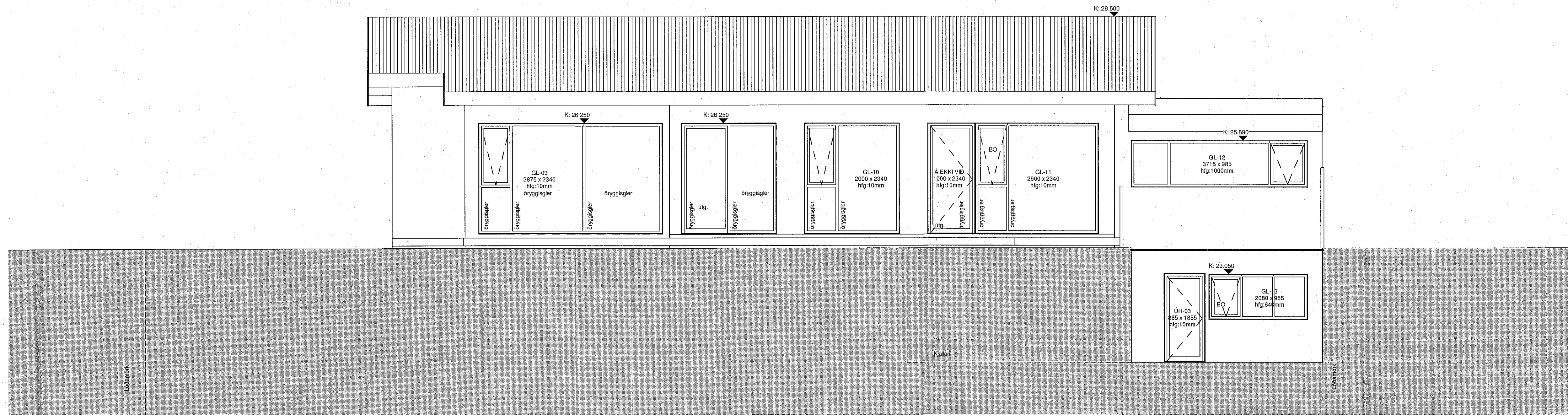
1 Útlit Suður VT 1:50
