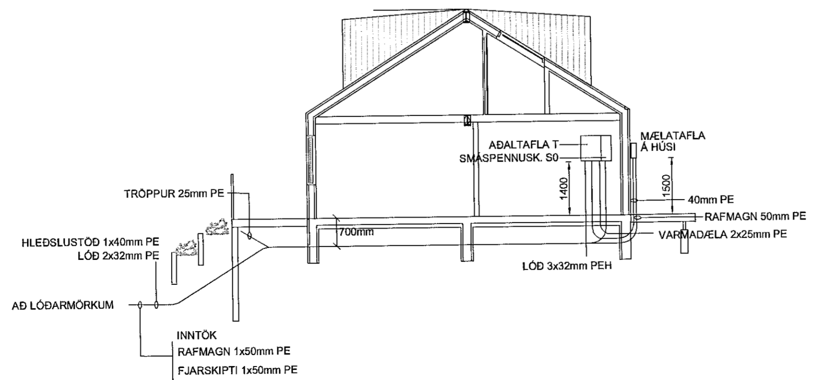
SNÍÐ A - A M 1:100
