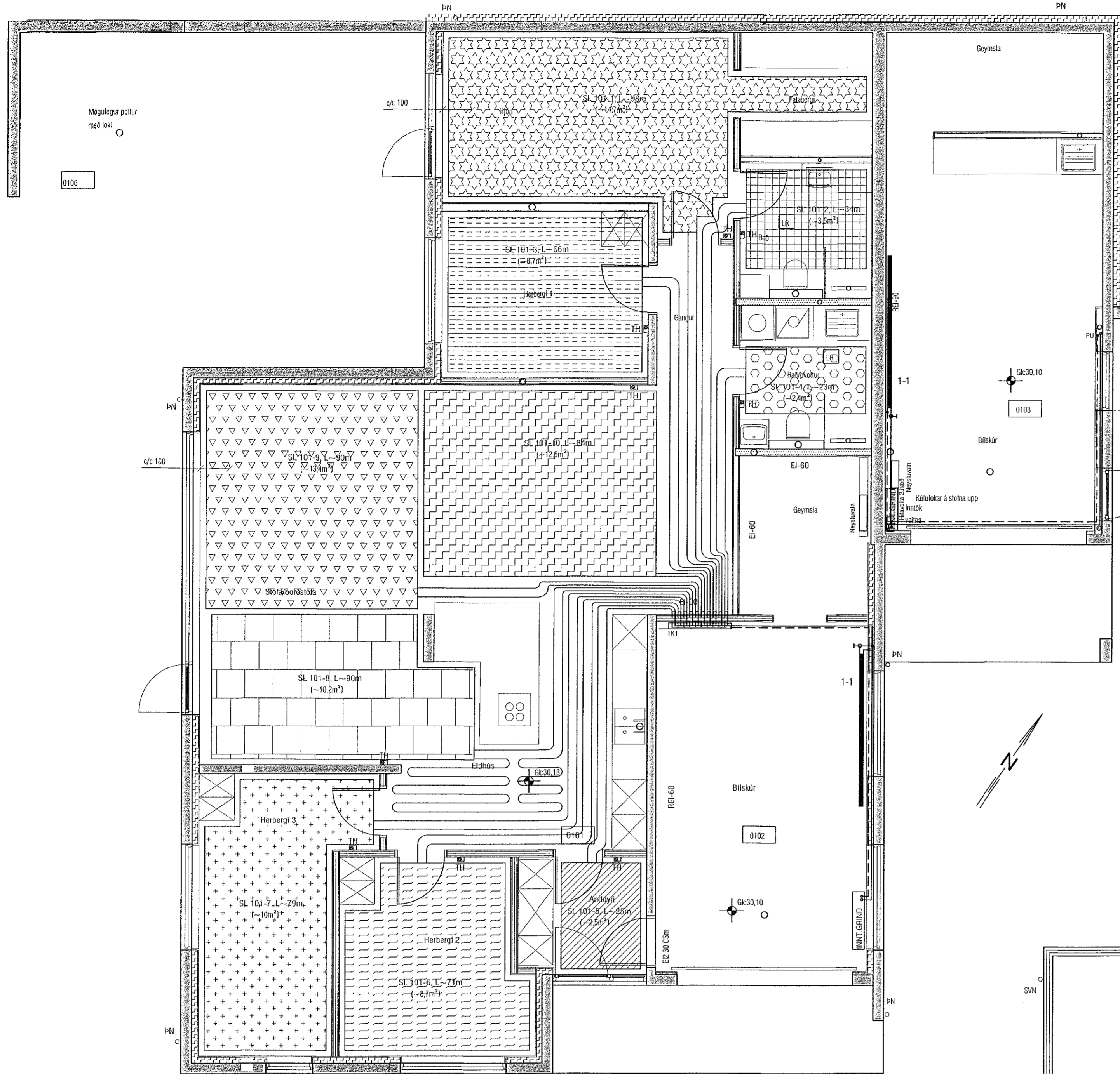
GRUNNMYND HITALAGNA 1. HÆÐ
