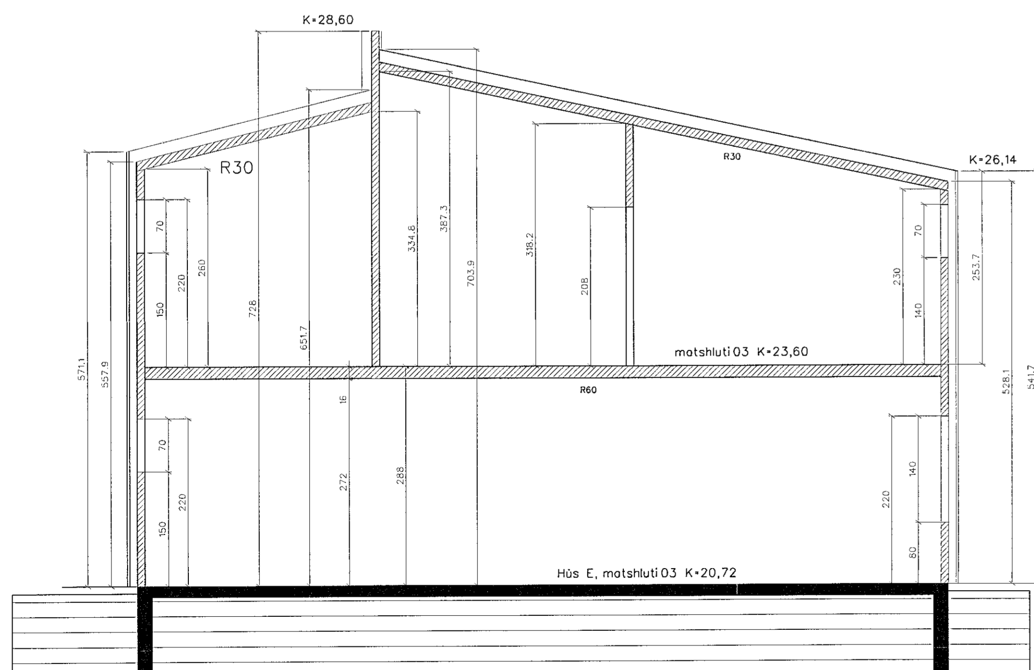
Hrauntunga 5E, einbýlishús. snid Snid B-B
