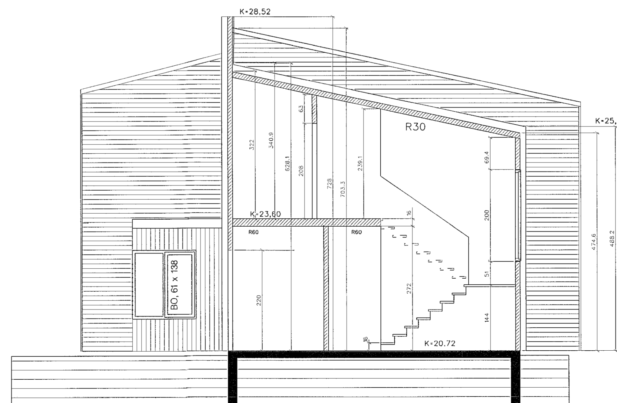
Hrauntunga 5E, einbýlishús. snid Snid C-C
