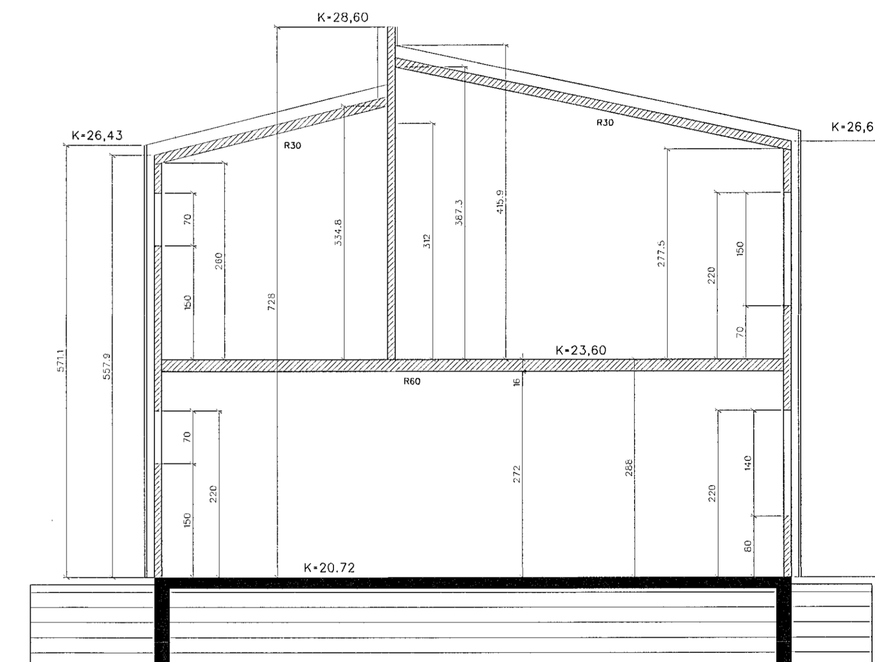
Hrauntunga 5E, einbýlishús. snid Snid A-A
