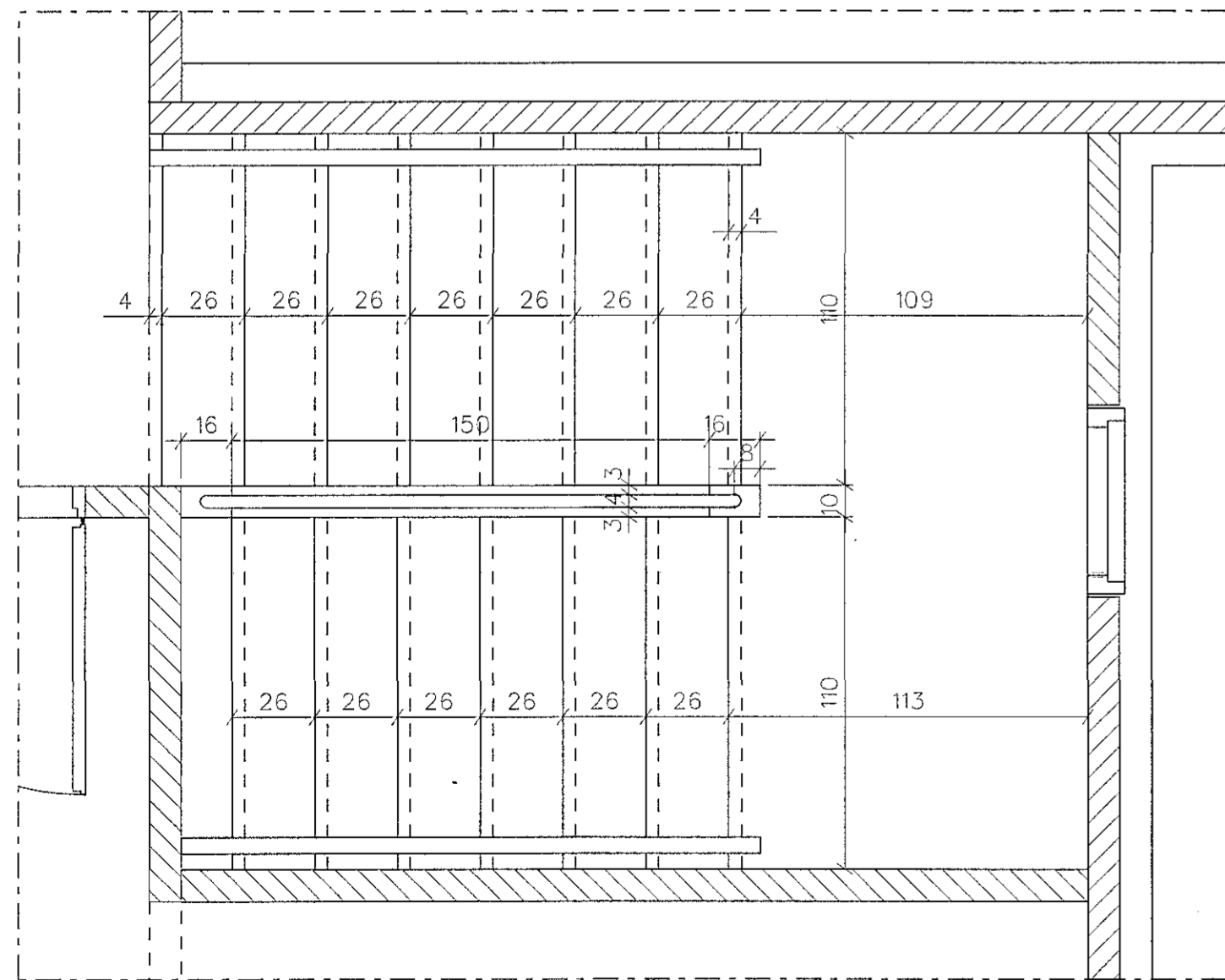
Hrauntunga 5, stigi, 2. hæð
