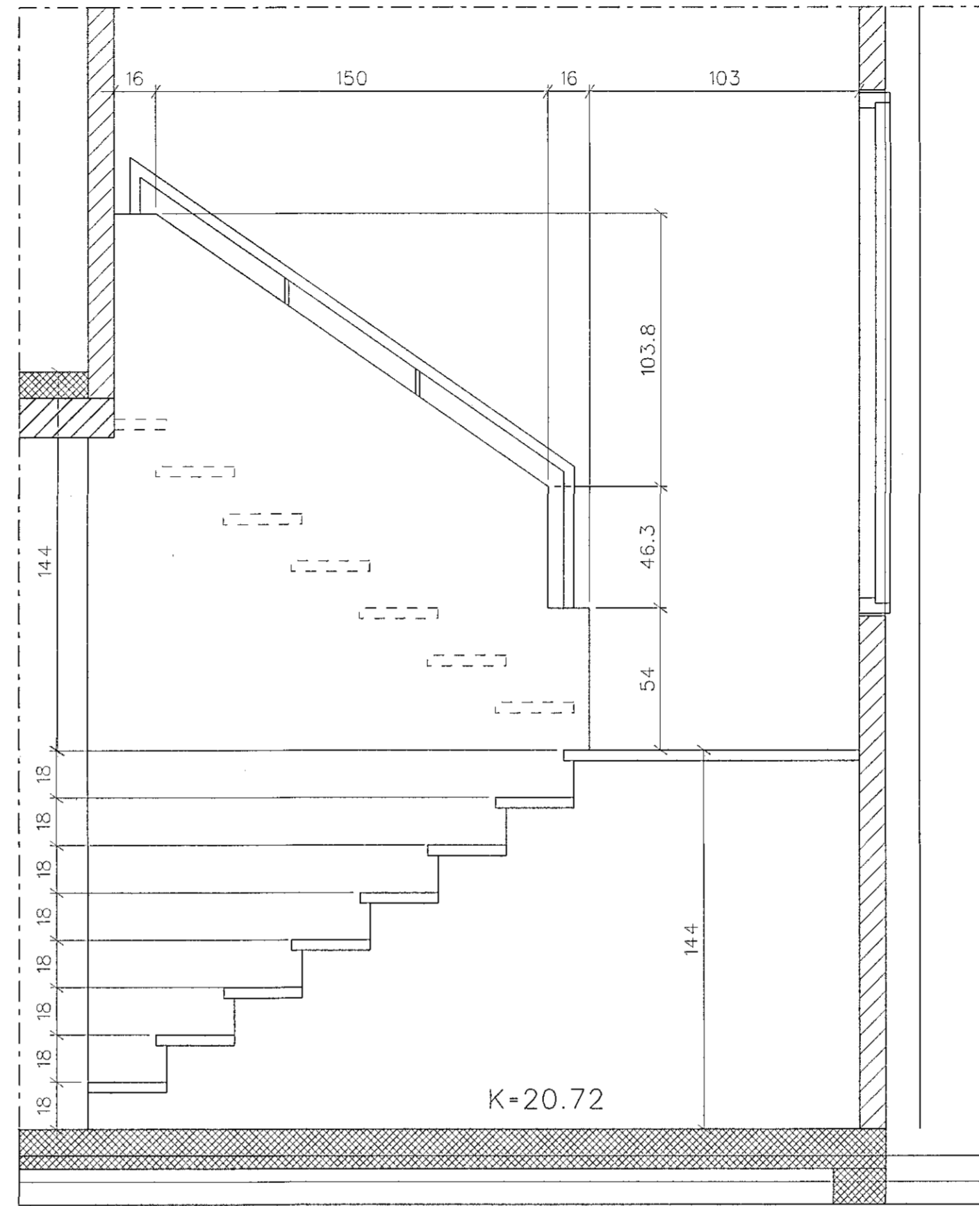
Hrauntunga 5, stigi, snið.
