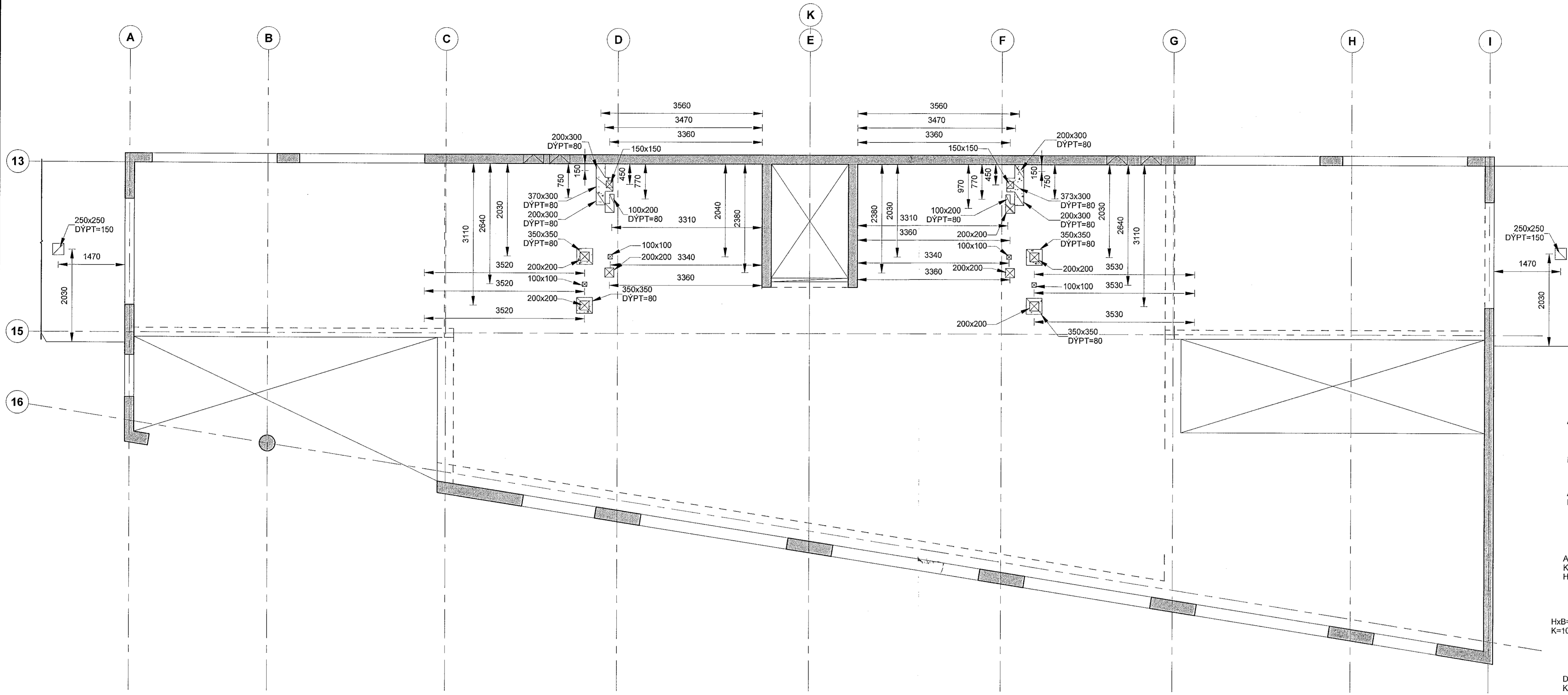
GRUNNMYND 2. HÆÐ GATAPLAN 1:50
