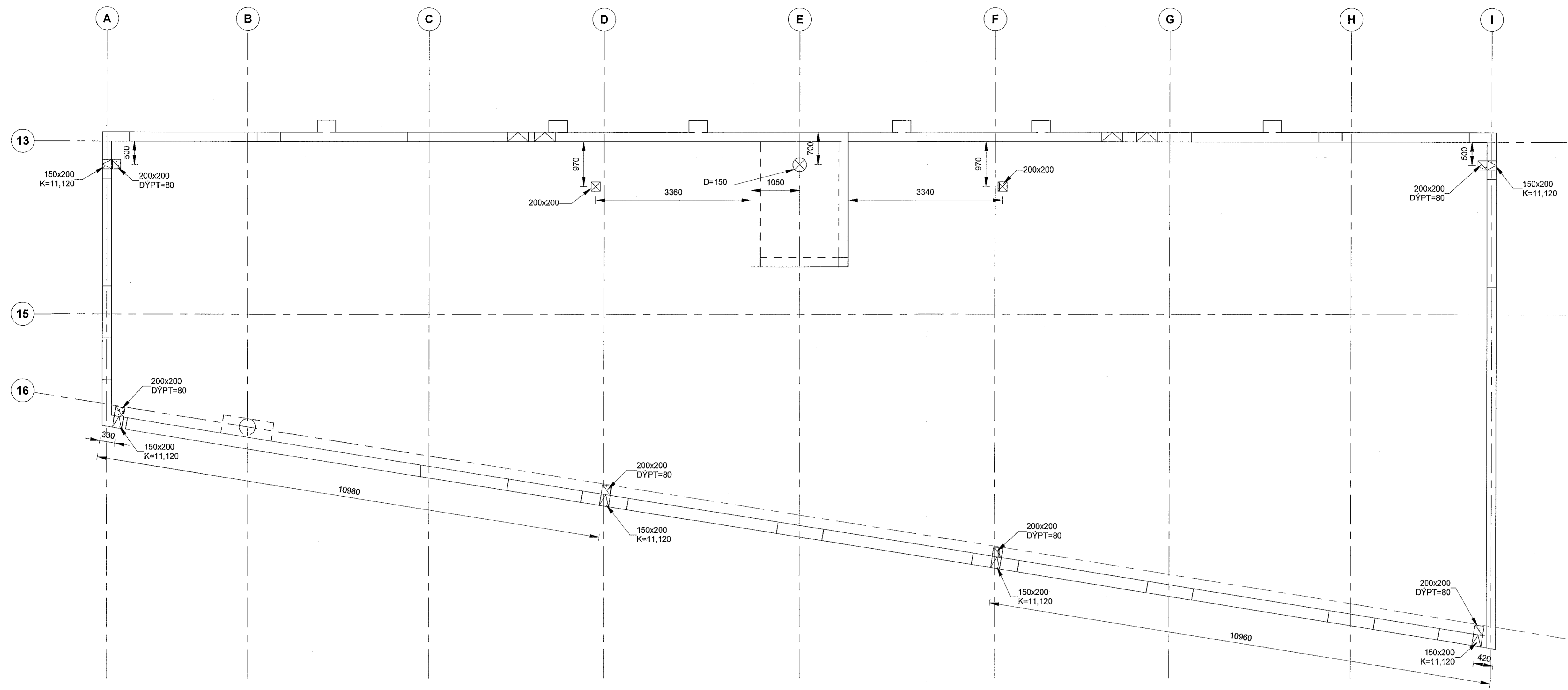
GRUNNMYND, 3. HÆÐ GATAPLAN 1:50
