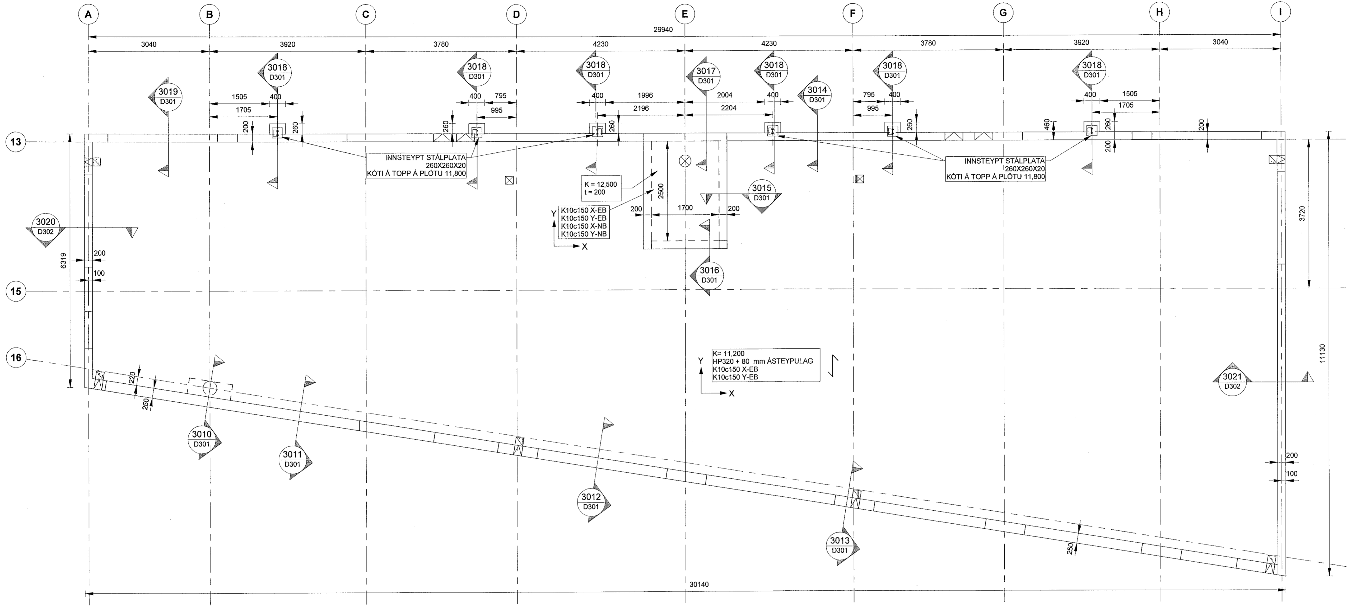
GRUNNMYND 3. HÆÐ 1:50
