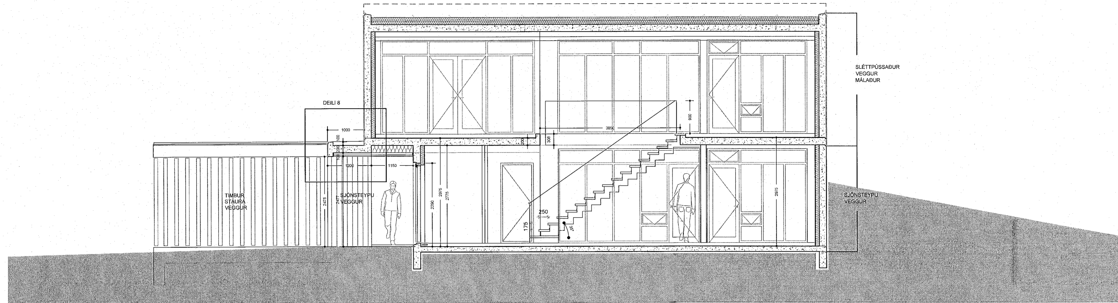
Snið A-A 1:50
