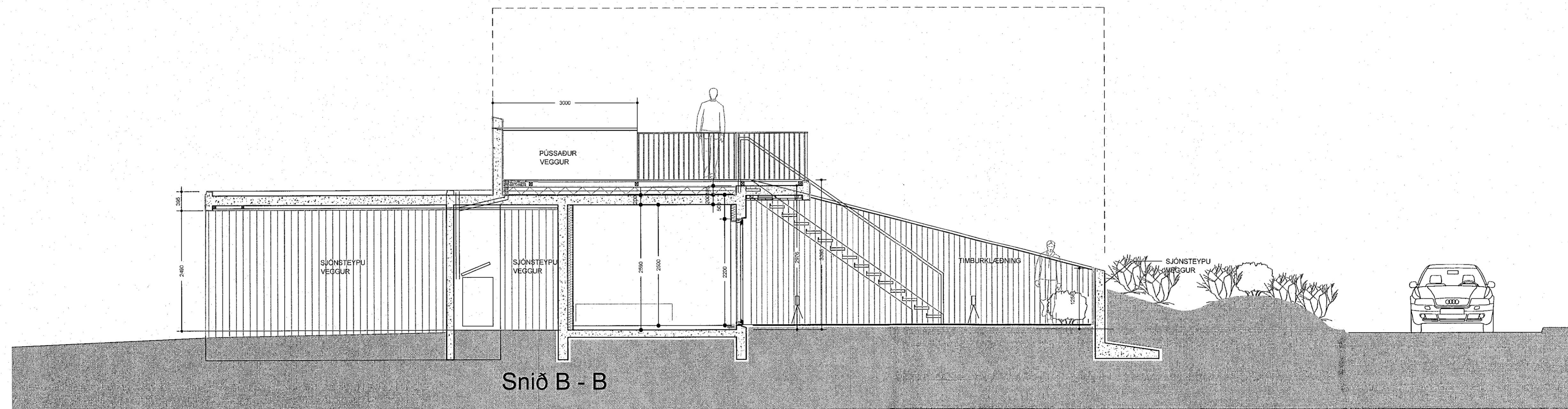
Snið B-B 1:50
