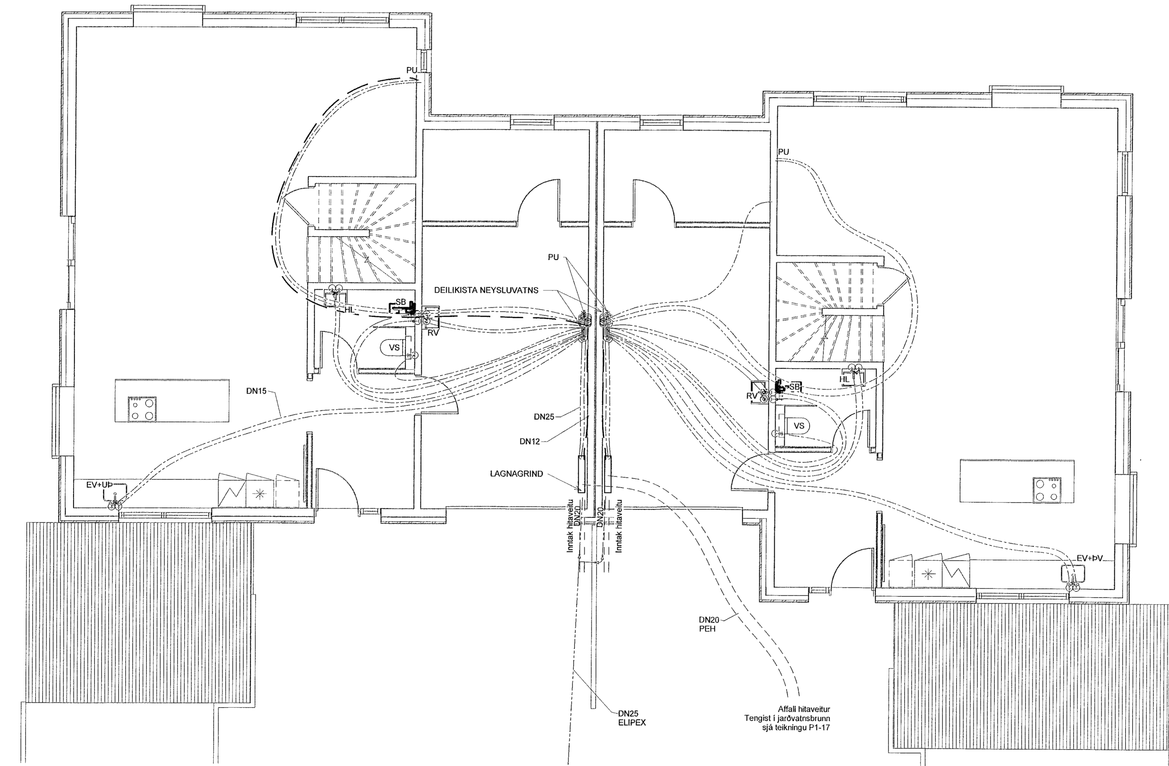
GRUNNMYND MKV.1:50
