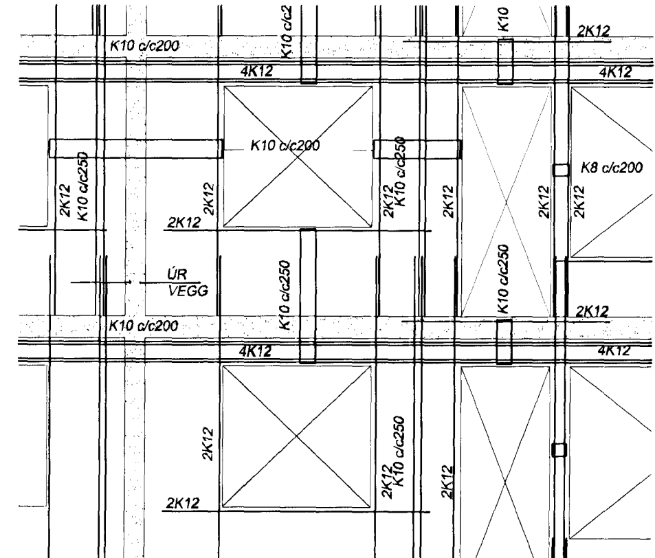
BENDING VEGGJA
