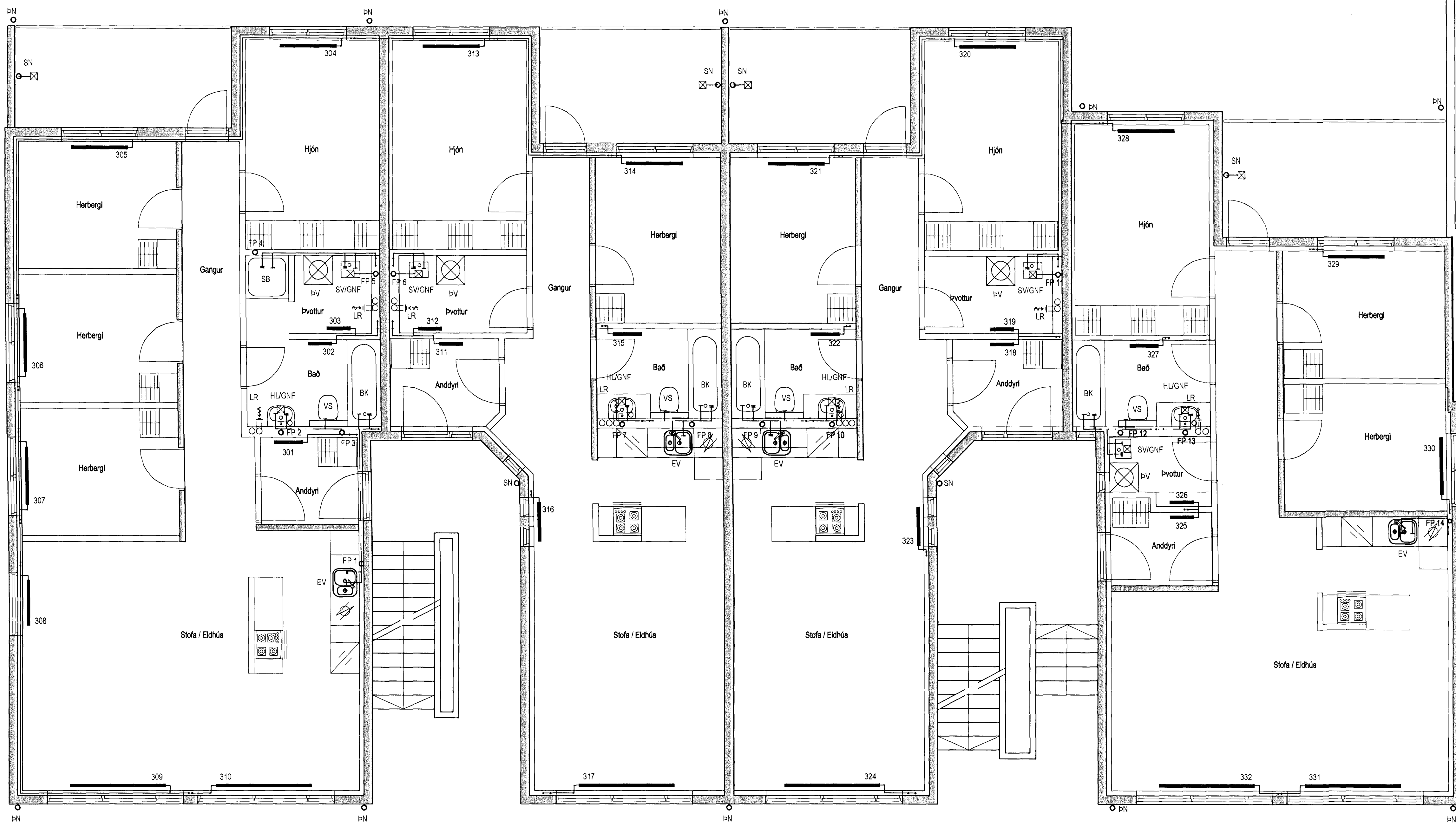
Lagnir 3. hæð, Grunnmynd 1:50
