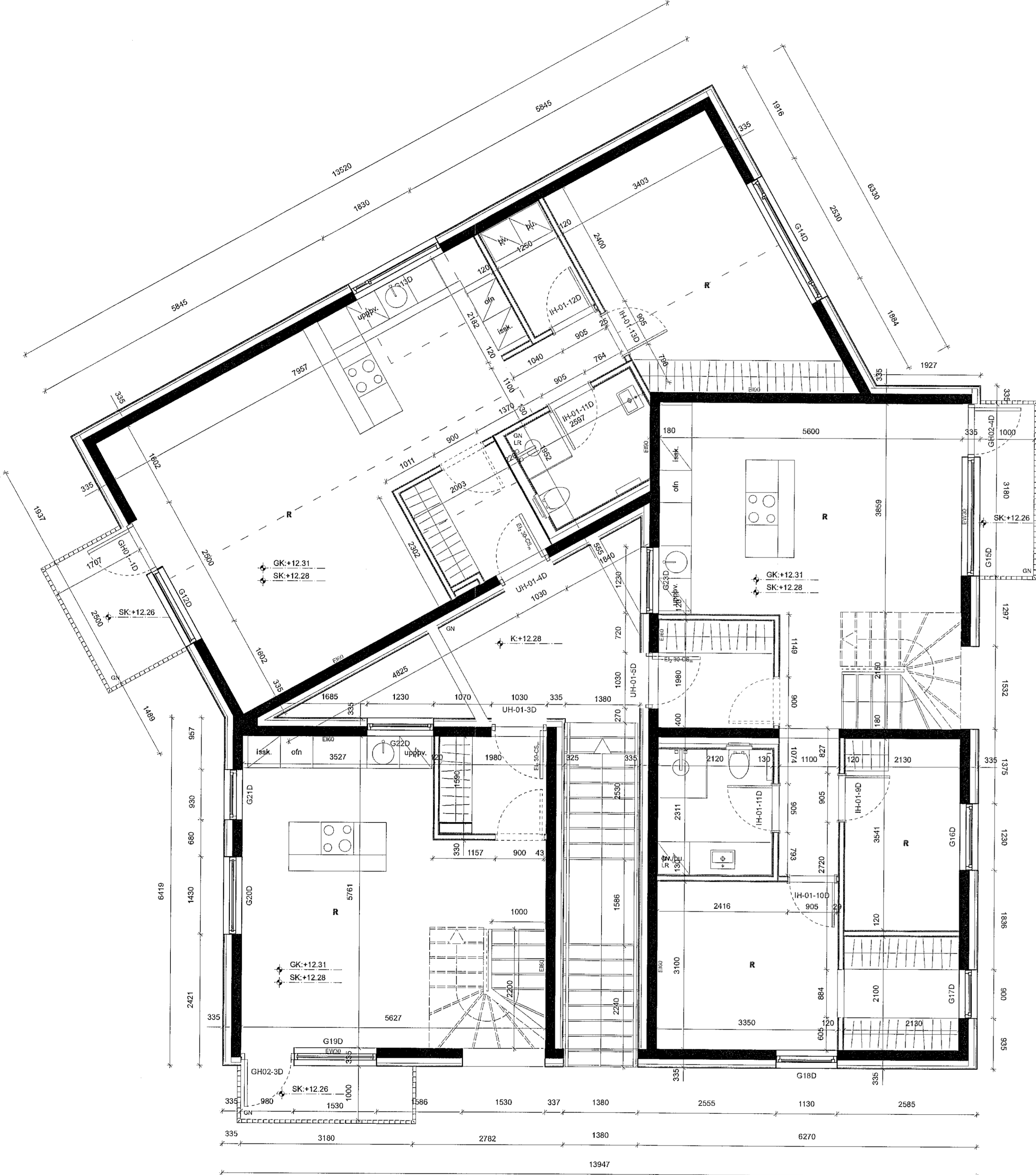
17 GRUNNMYND +3 (D-HÚS) Skali: 1:50
