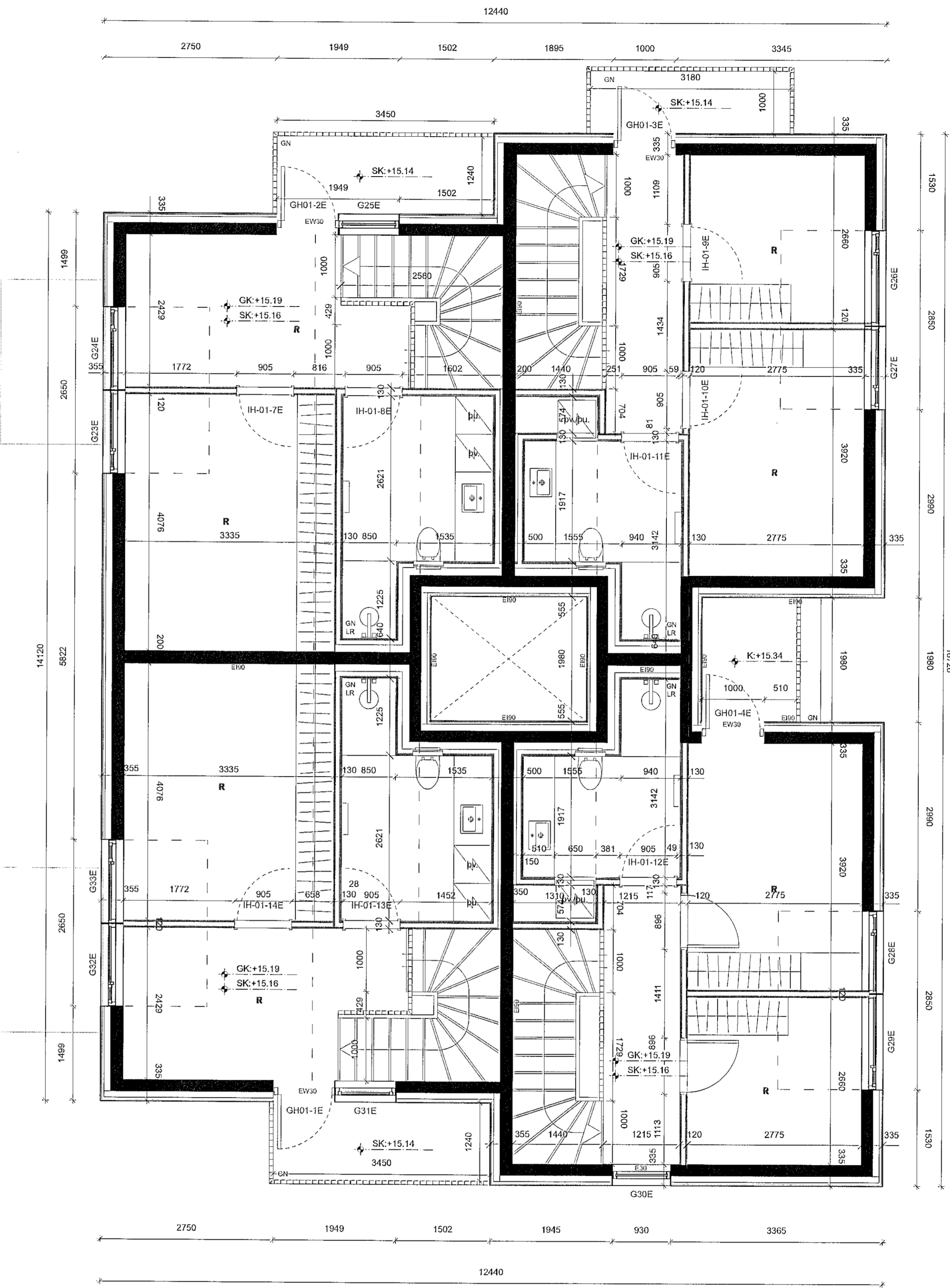
24 GRUNNMYND +4 (E-HÚS) Skali: 1:50
