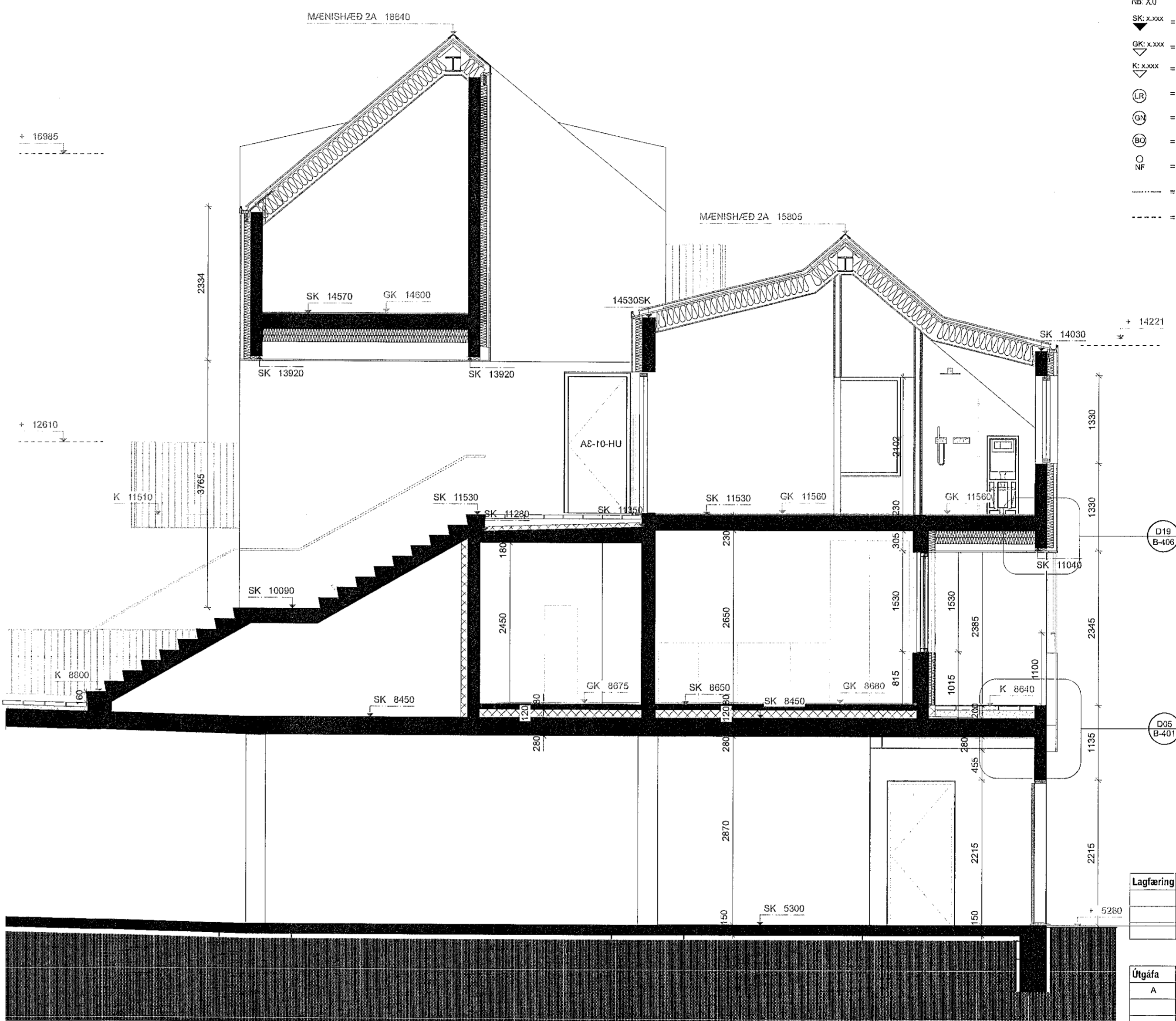
A2 SNEIDING A2 Skali: 1:50
