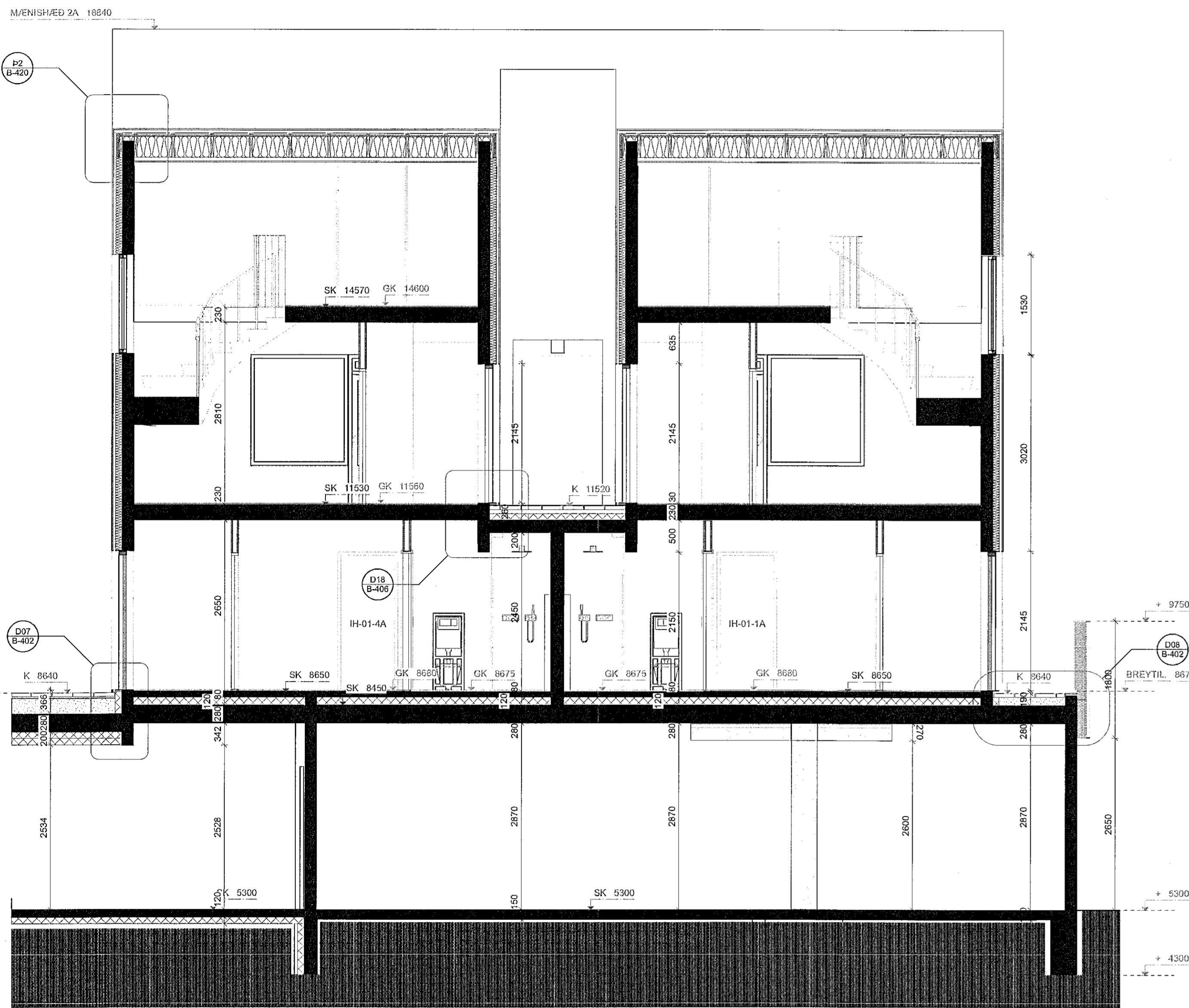
A1 SNEIDING A1 Skali: 1:50
