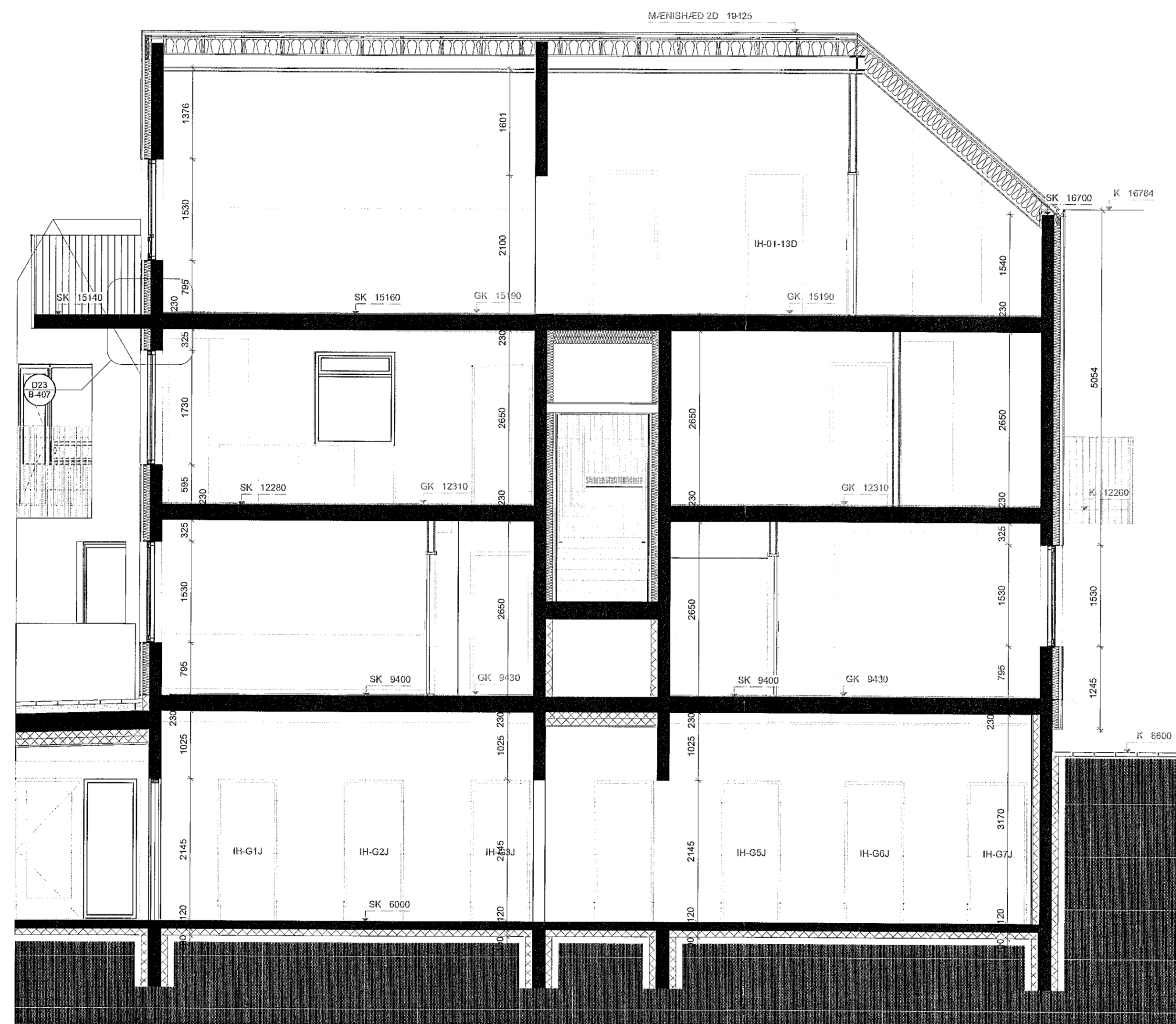
D2 SNEIÐING D2 Skali: 1:50
