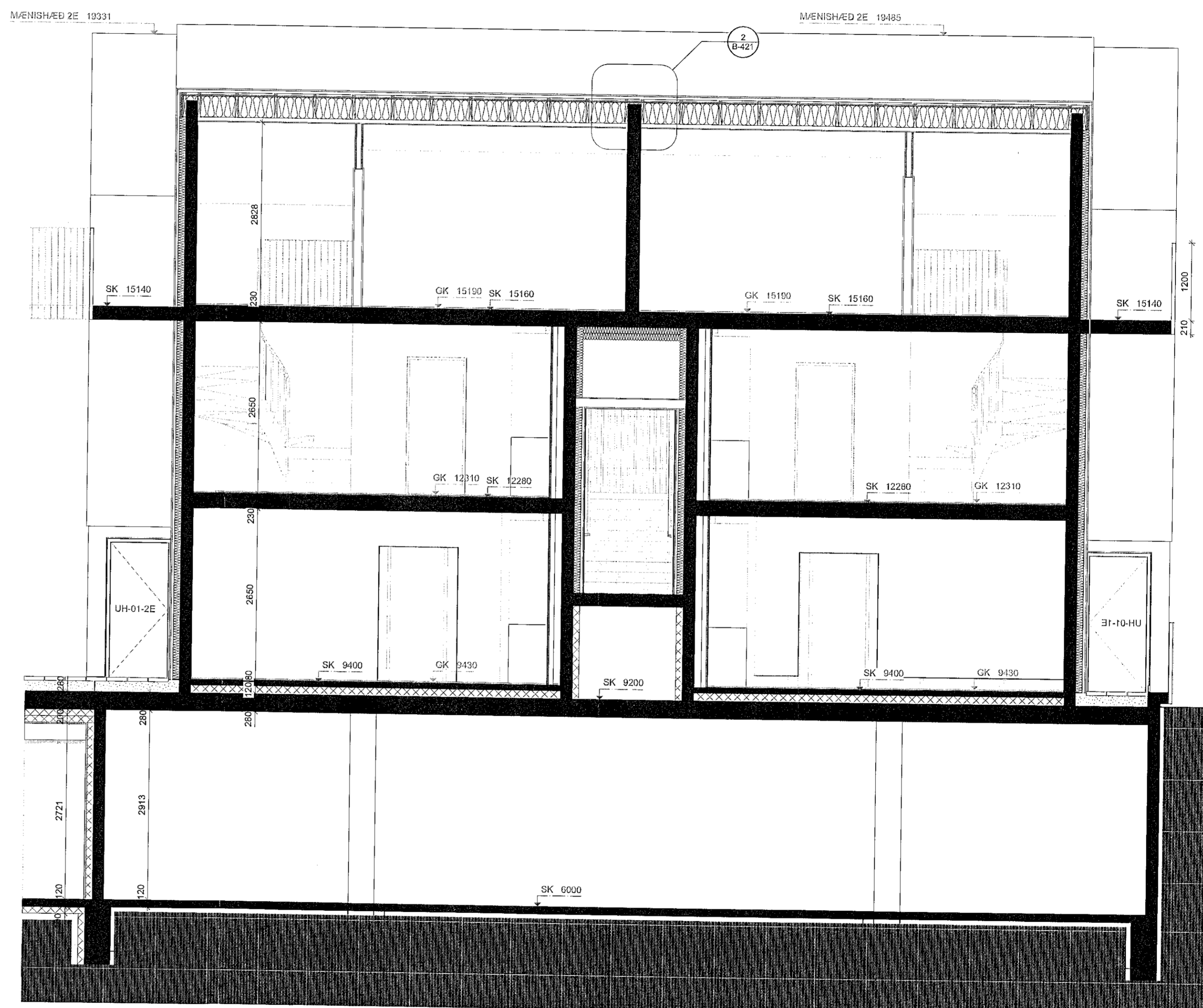
E2 SNEIDING E2 Skali: 1:50
