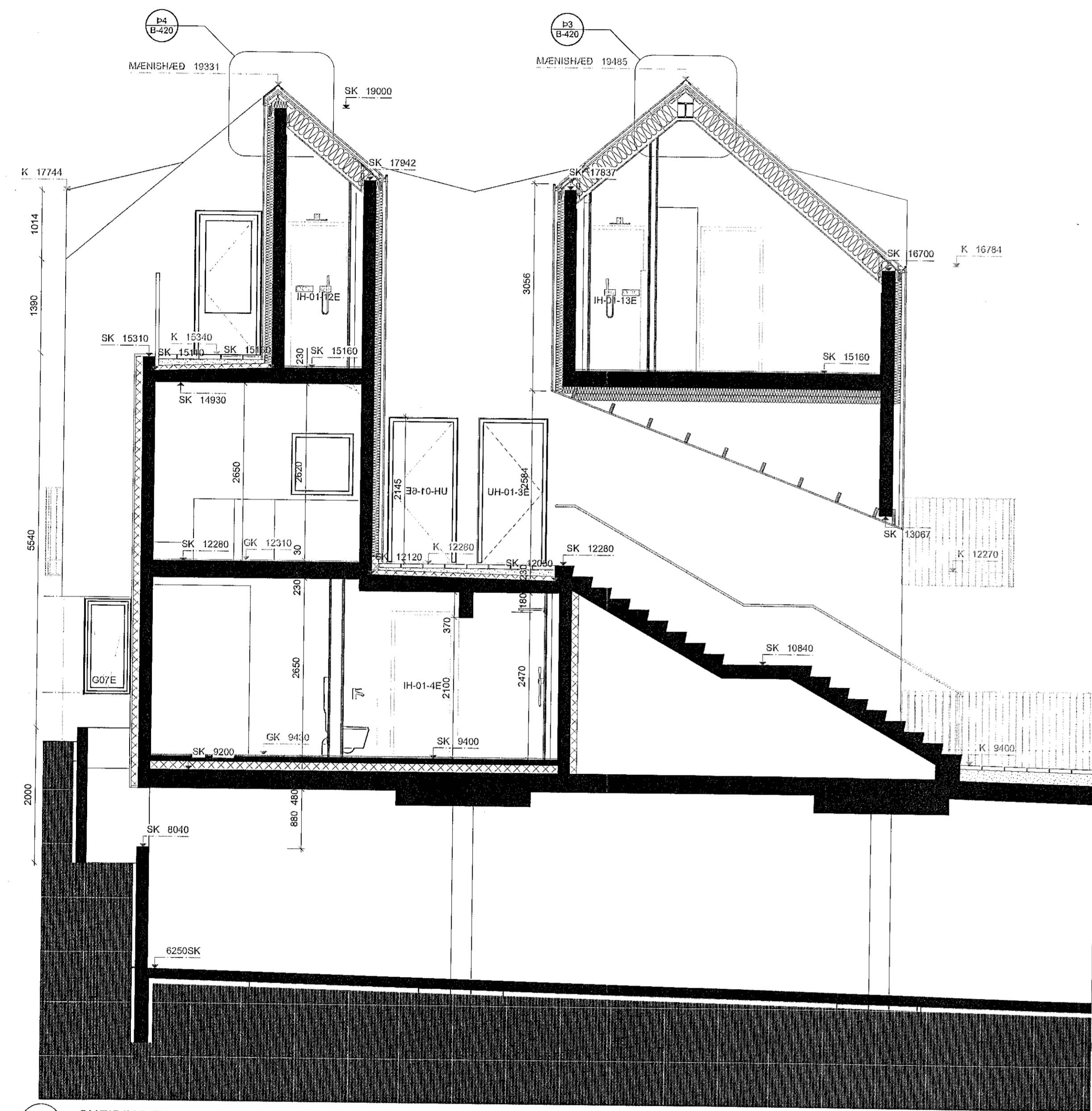
E1 SNEIDING E1 Skali: 1:50
