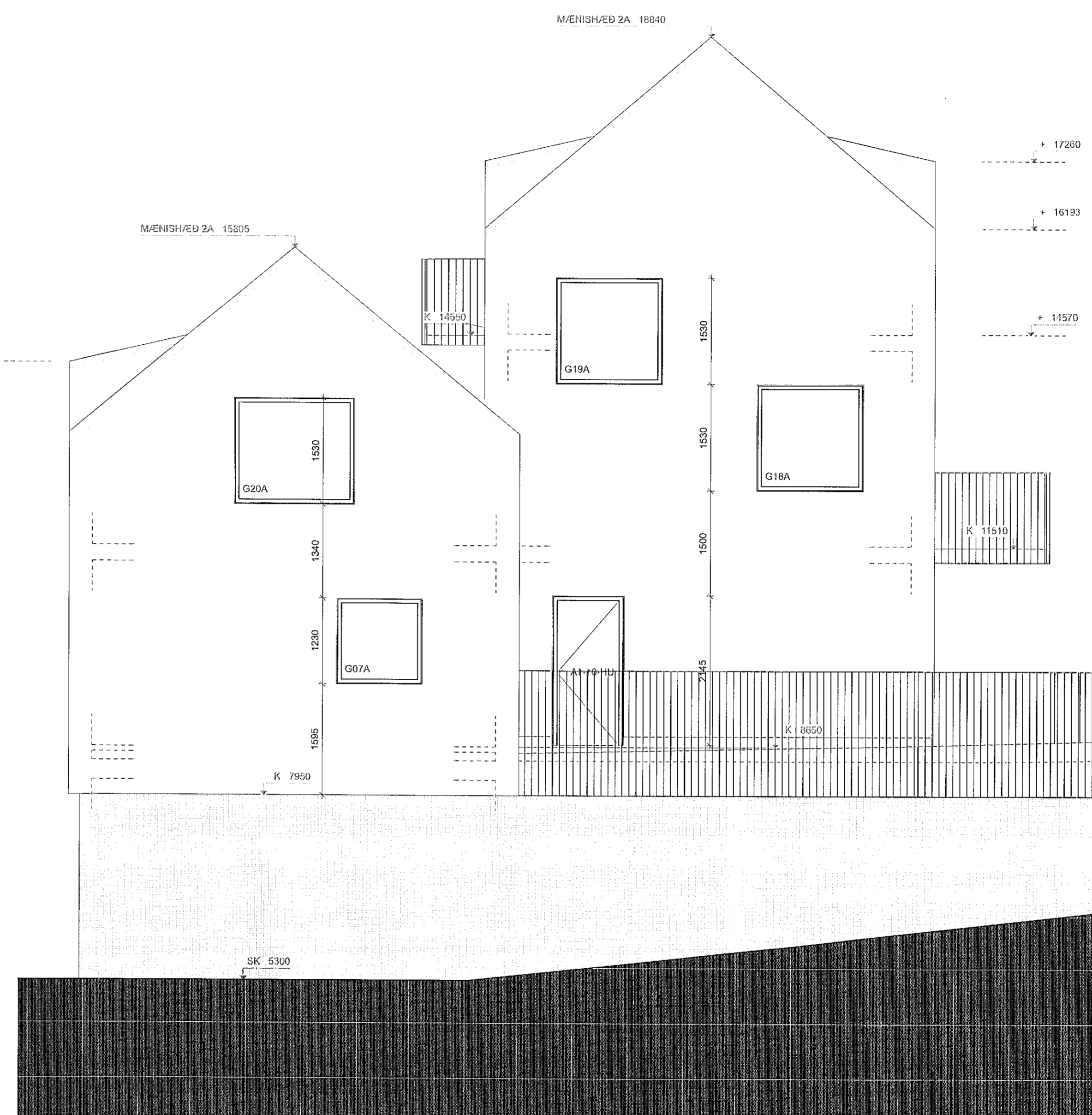
2 ÚTLIT SUÐUR Skali: 1:50
