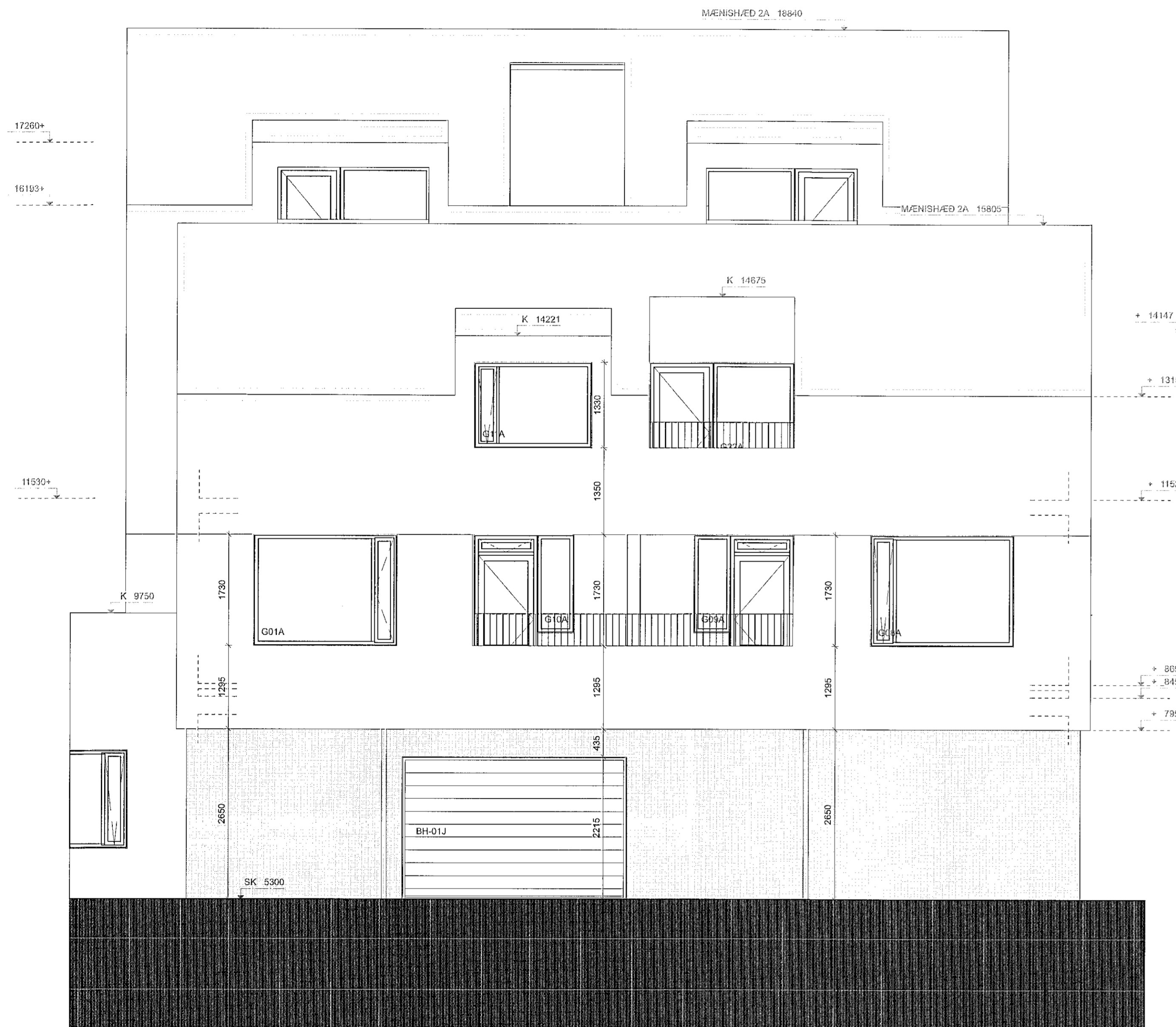
1 ÚTLIT VESTUR Skali: 1:50
