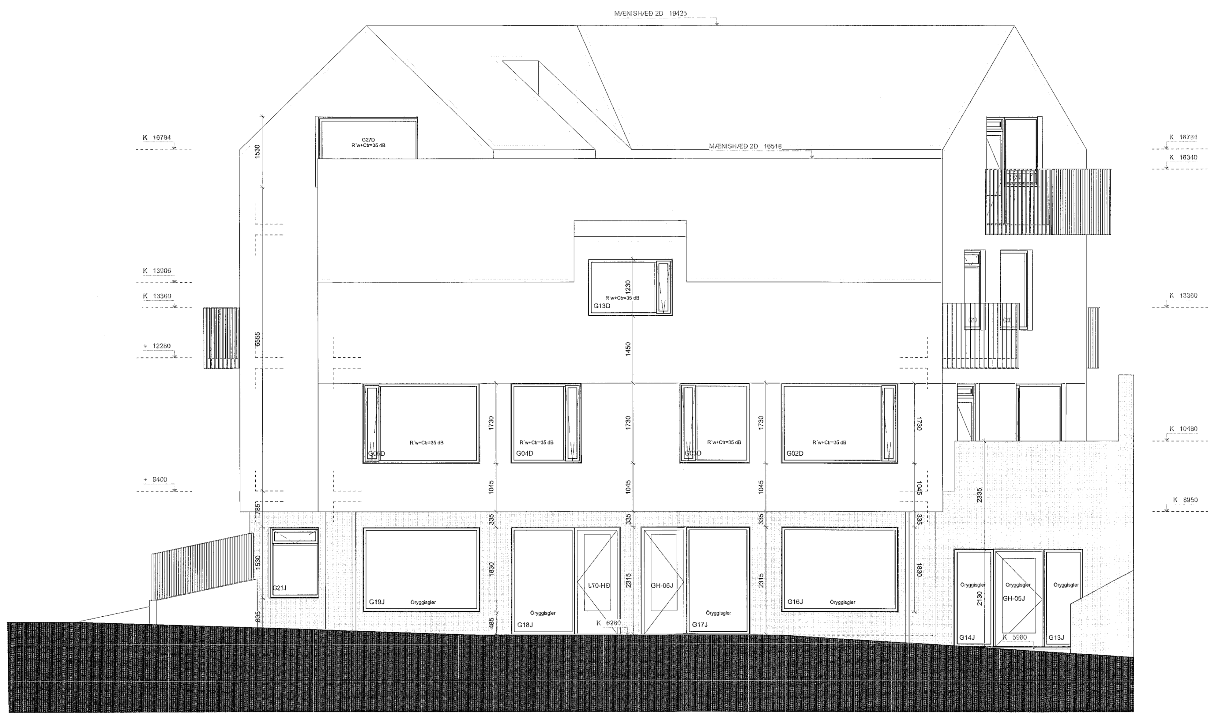
2 2D ÚTLIT NORÐUR Skali: 1:50
