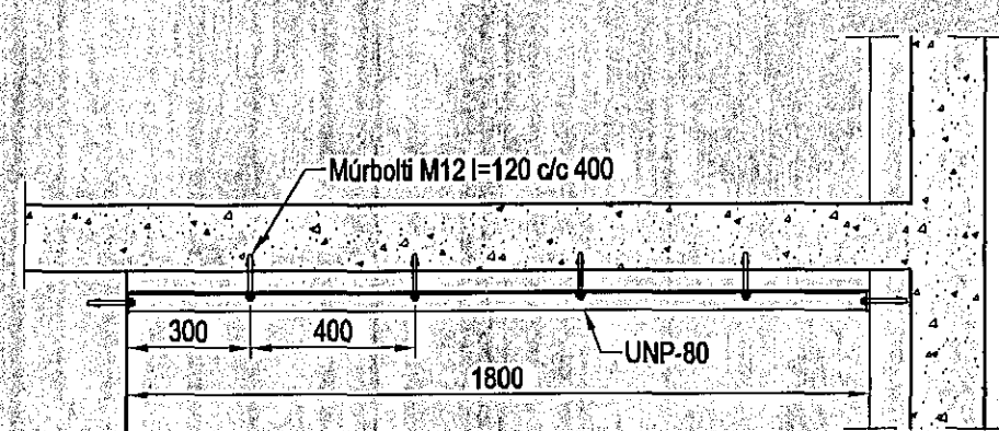
Gat í burðarvegg, Snið, 1:20
