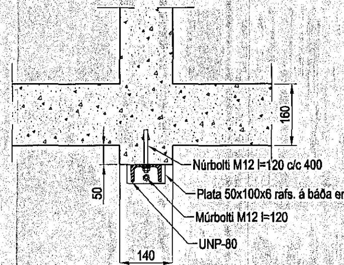
Gat í burðarvegg, Snið, 1:10
