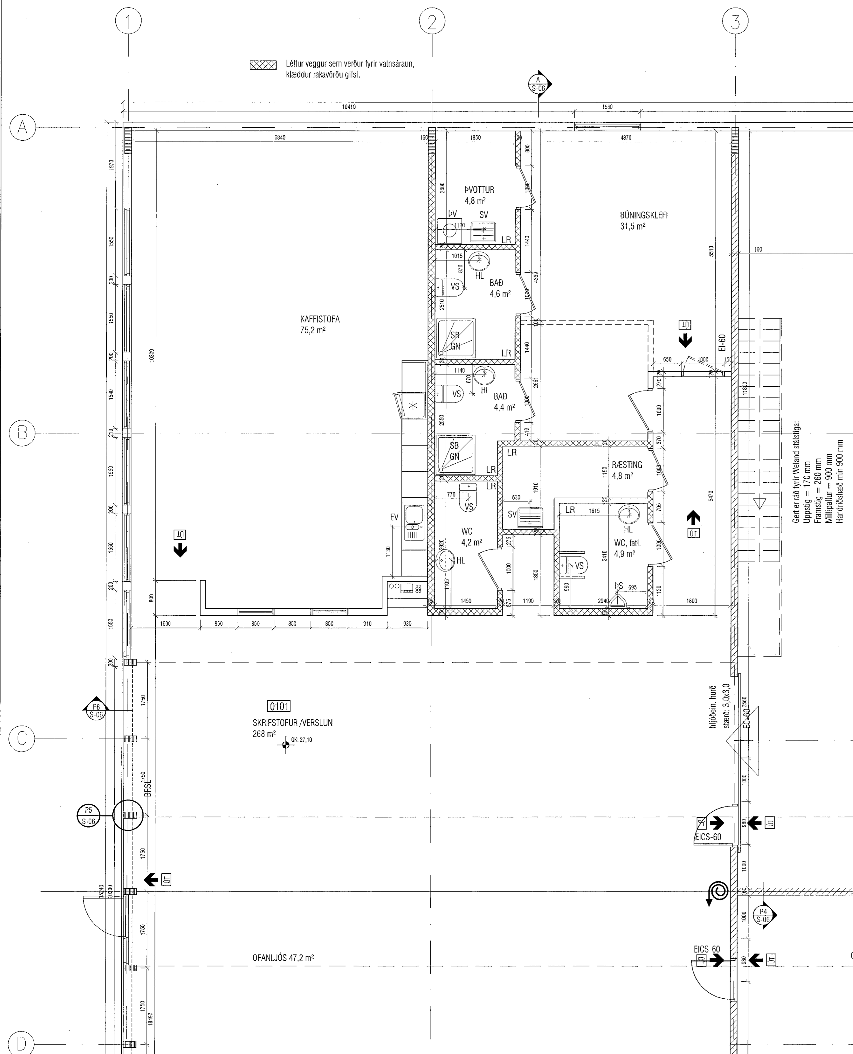
NORÐVESTURHLUTI Mkv. 1/50
