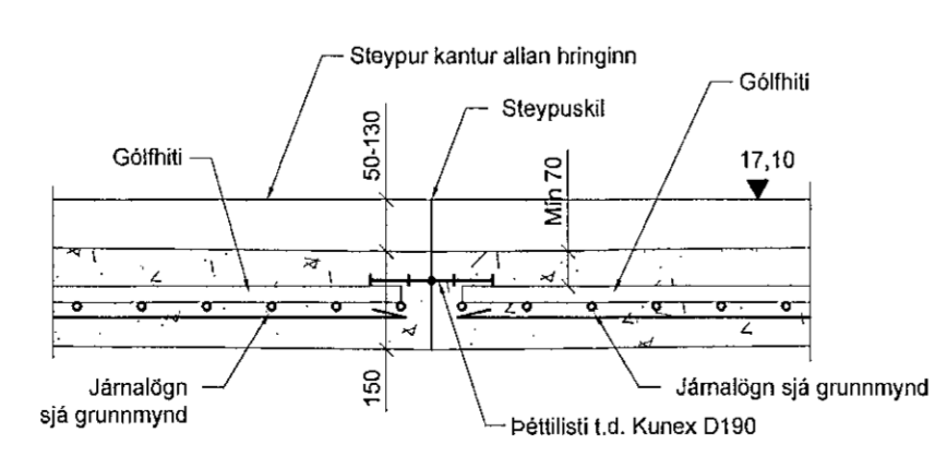
Snið í gólfhita við stöypuski
