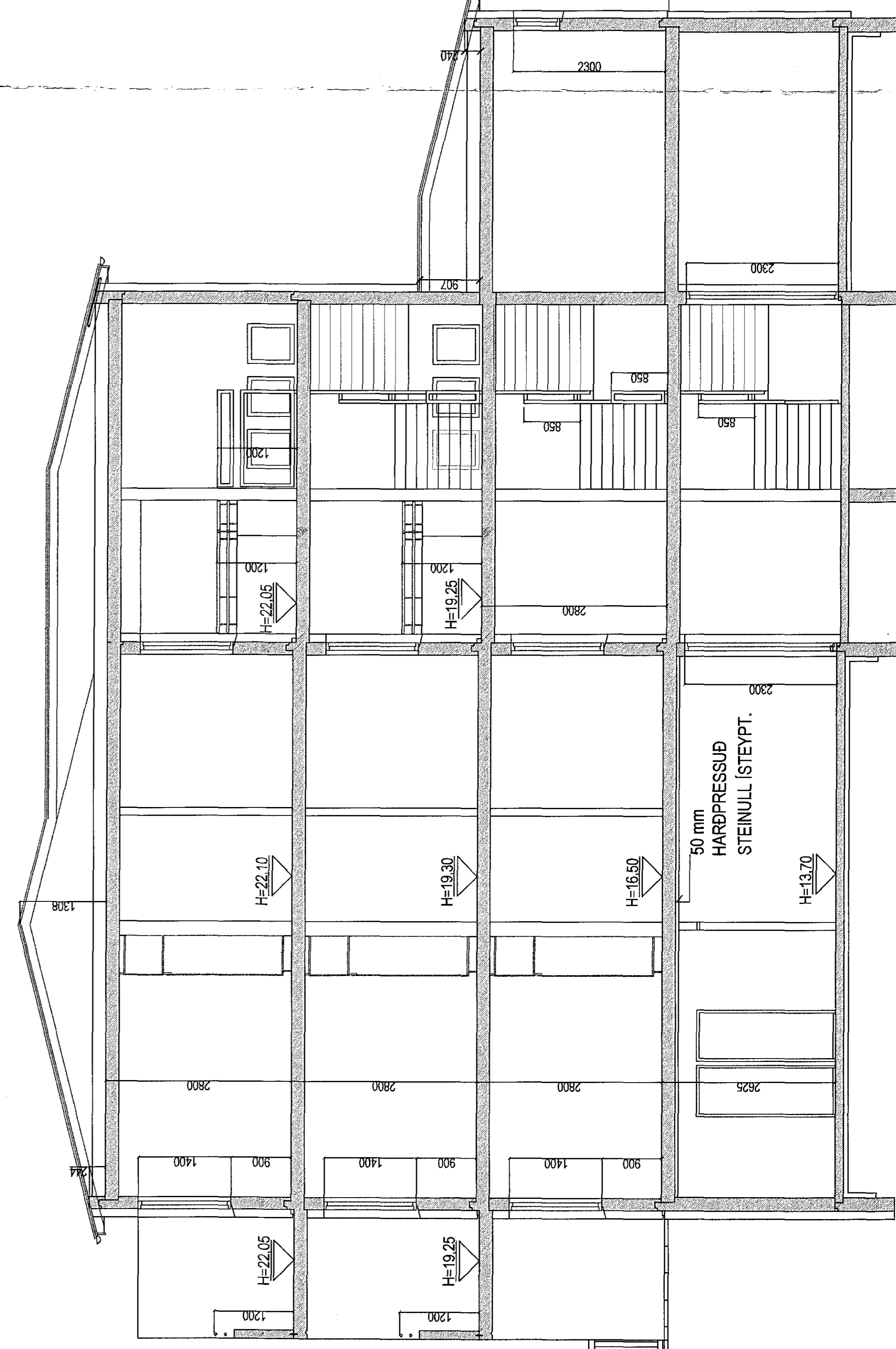
SNID B-B. MKV. 1:50.
