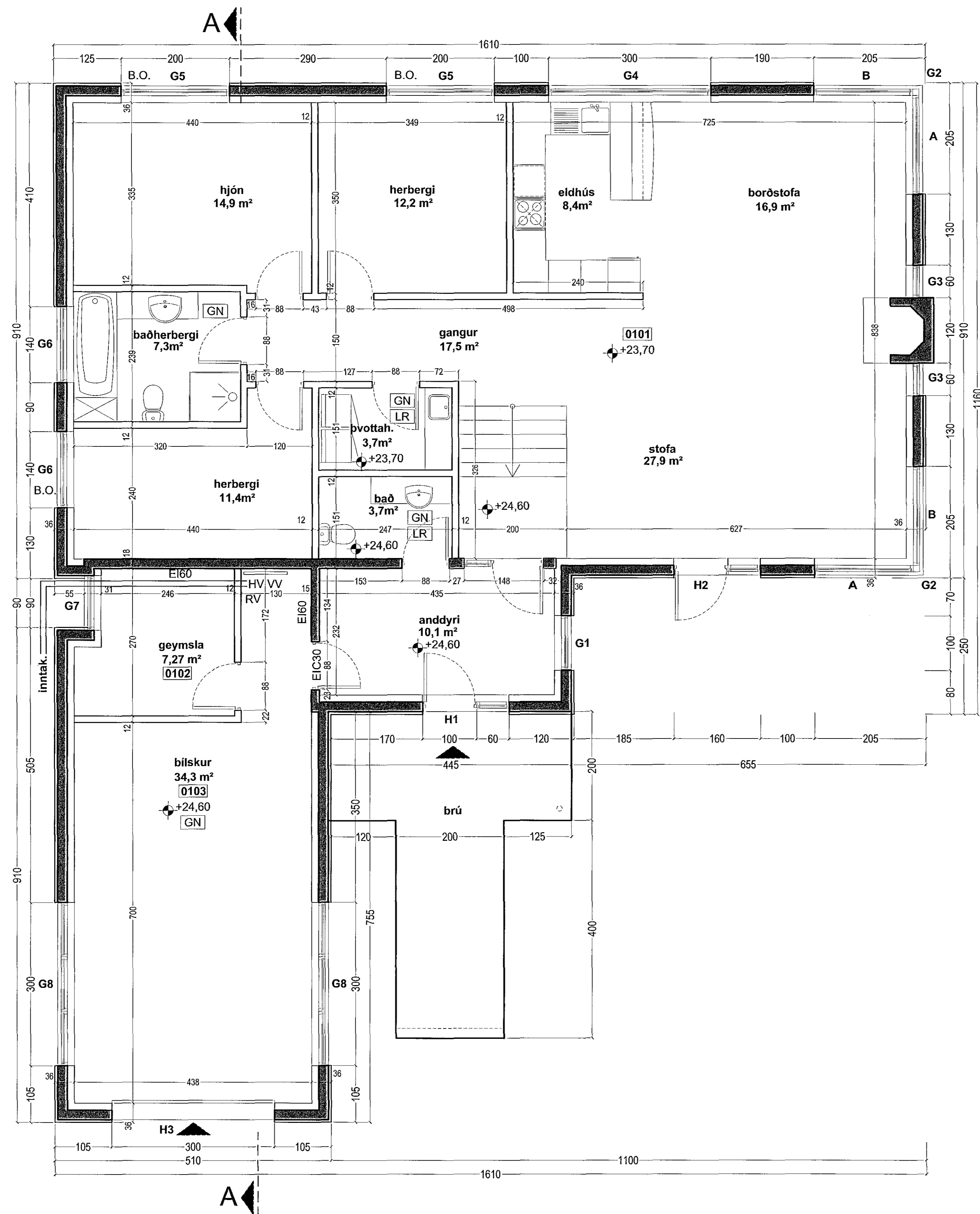
GRUNNMYND 1:50
