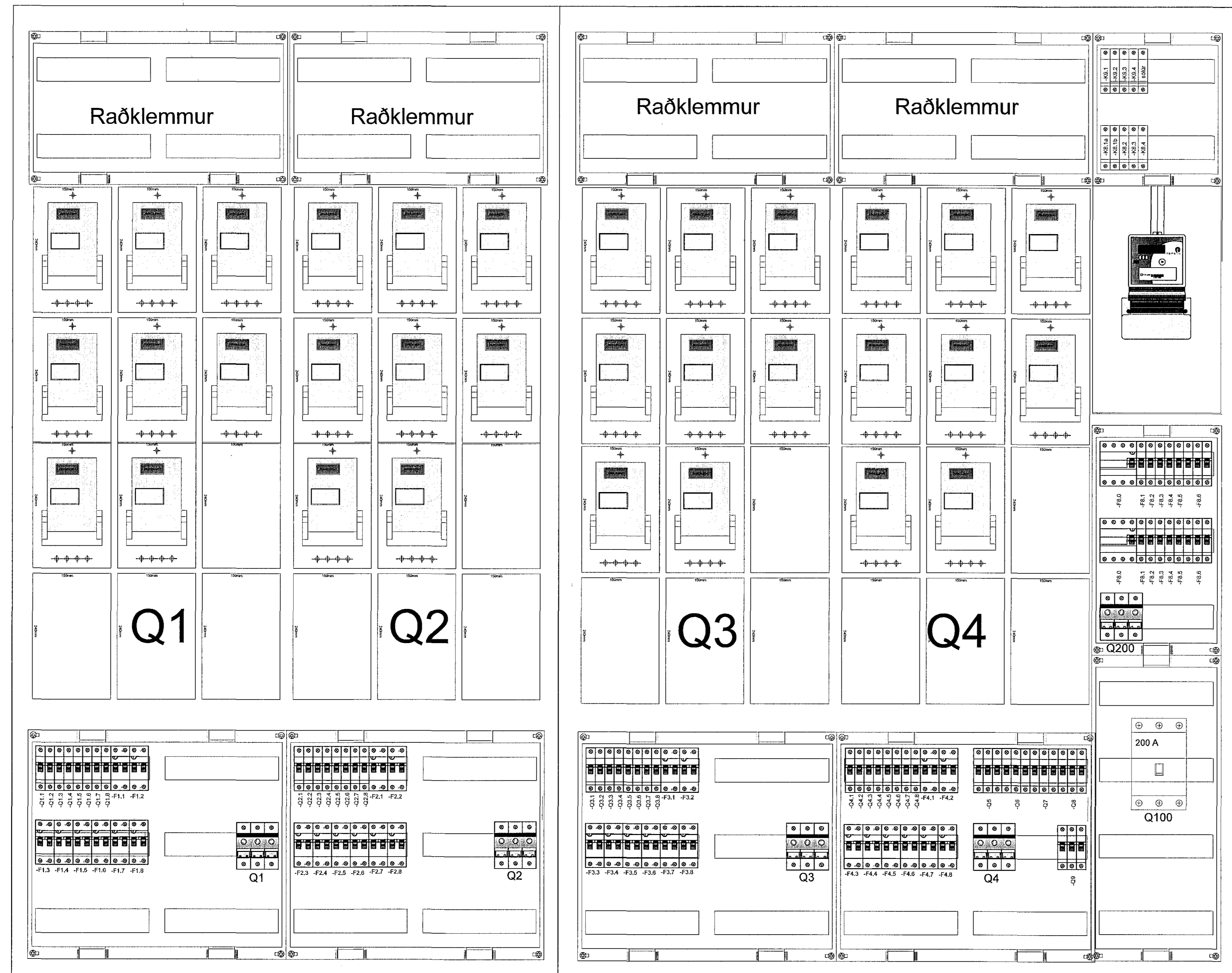
ADALTAFLA T.0 : STÆRÐ ca. 2350 X 1850 X 275 mm
