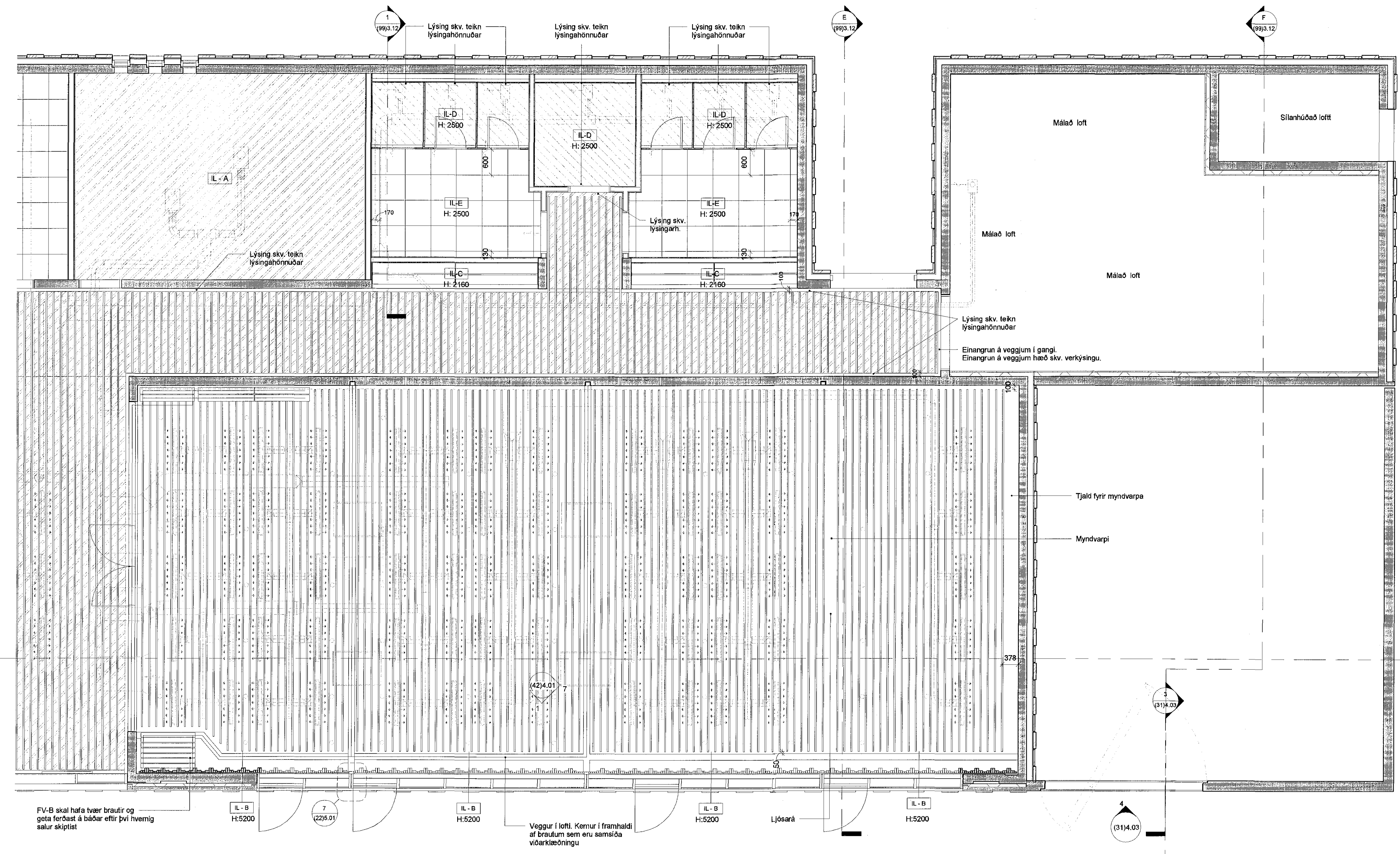
1 (35) Loftaplan 1. hæð - Svæði B 1 : 50
