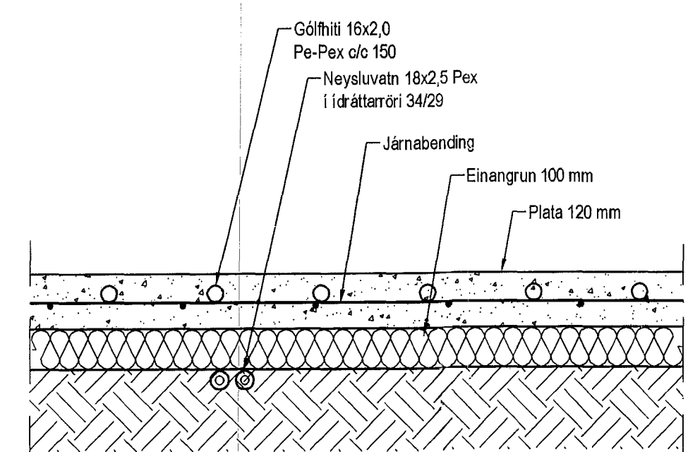
Hita- og vatnslagnir, Sníð í botnplötu bílageymslu, 1:10
