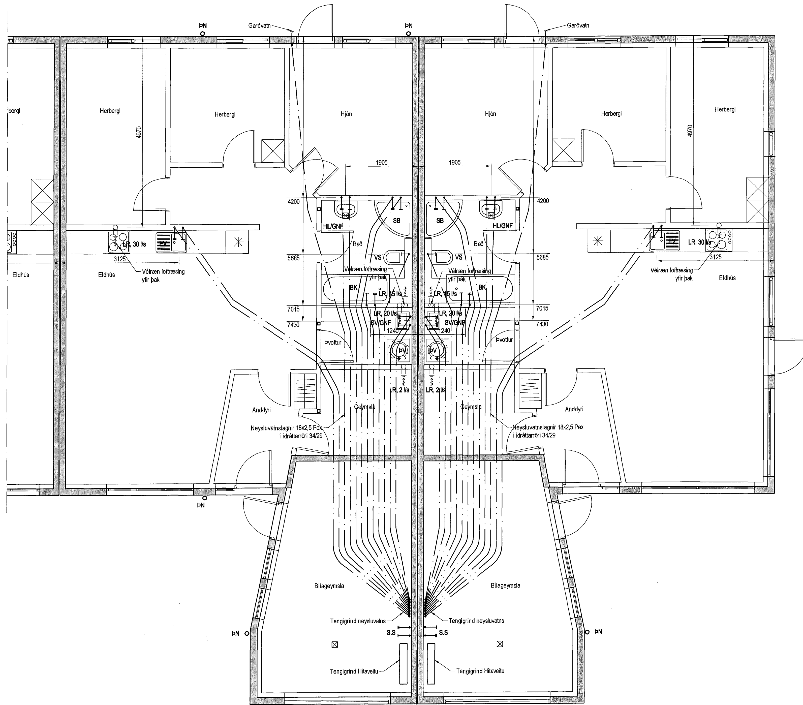
Neysluvatnslagnir 1. hæð, 1:50
