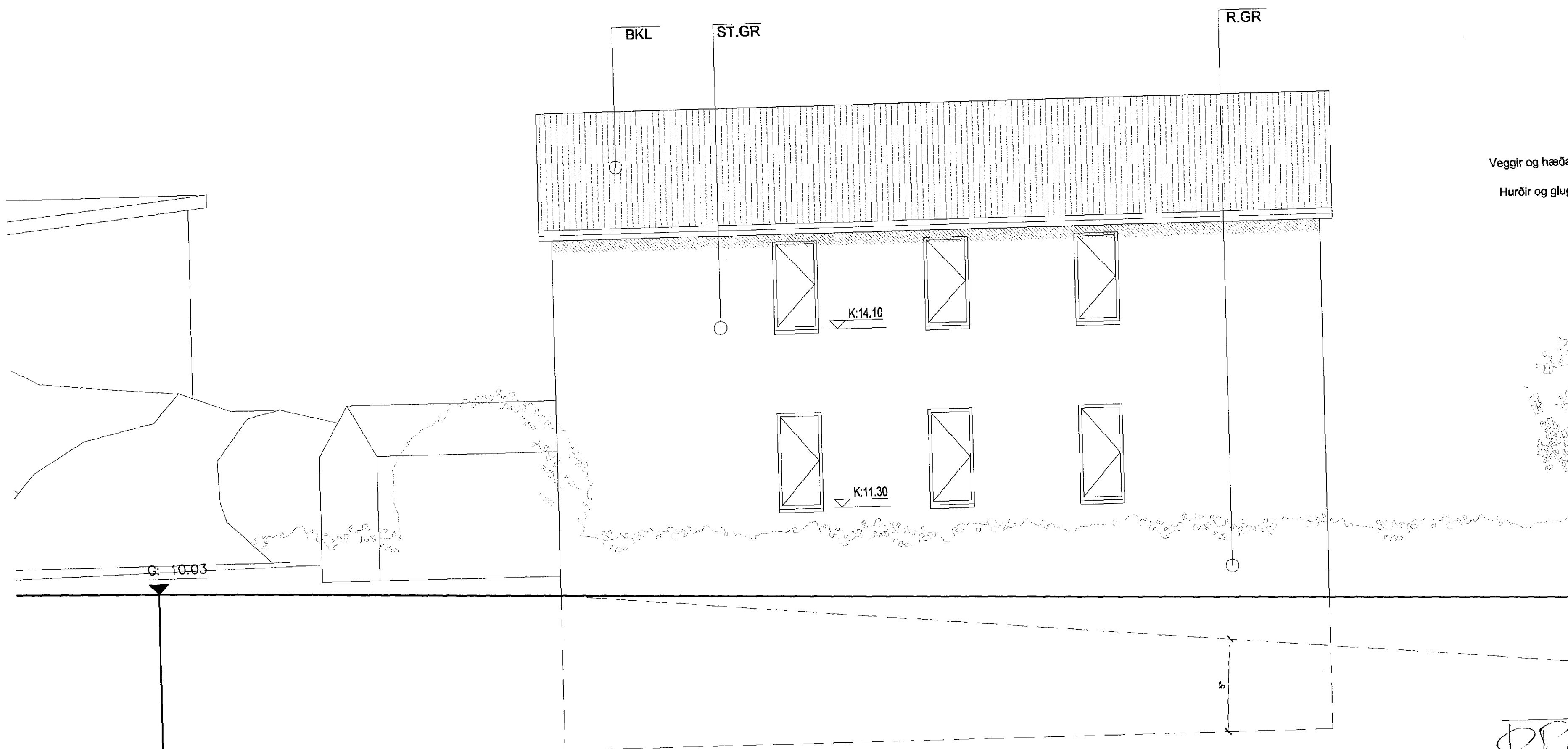
Ásýnd suð-vestur mkv. 1:50
