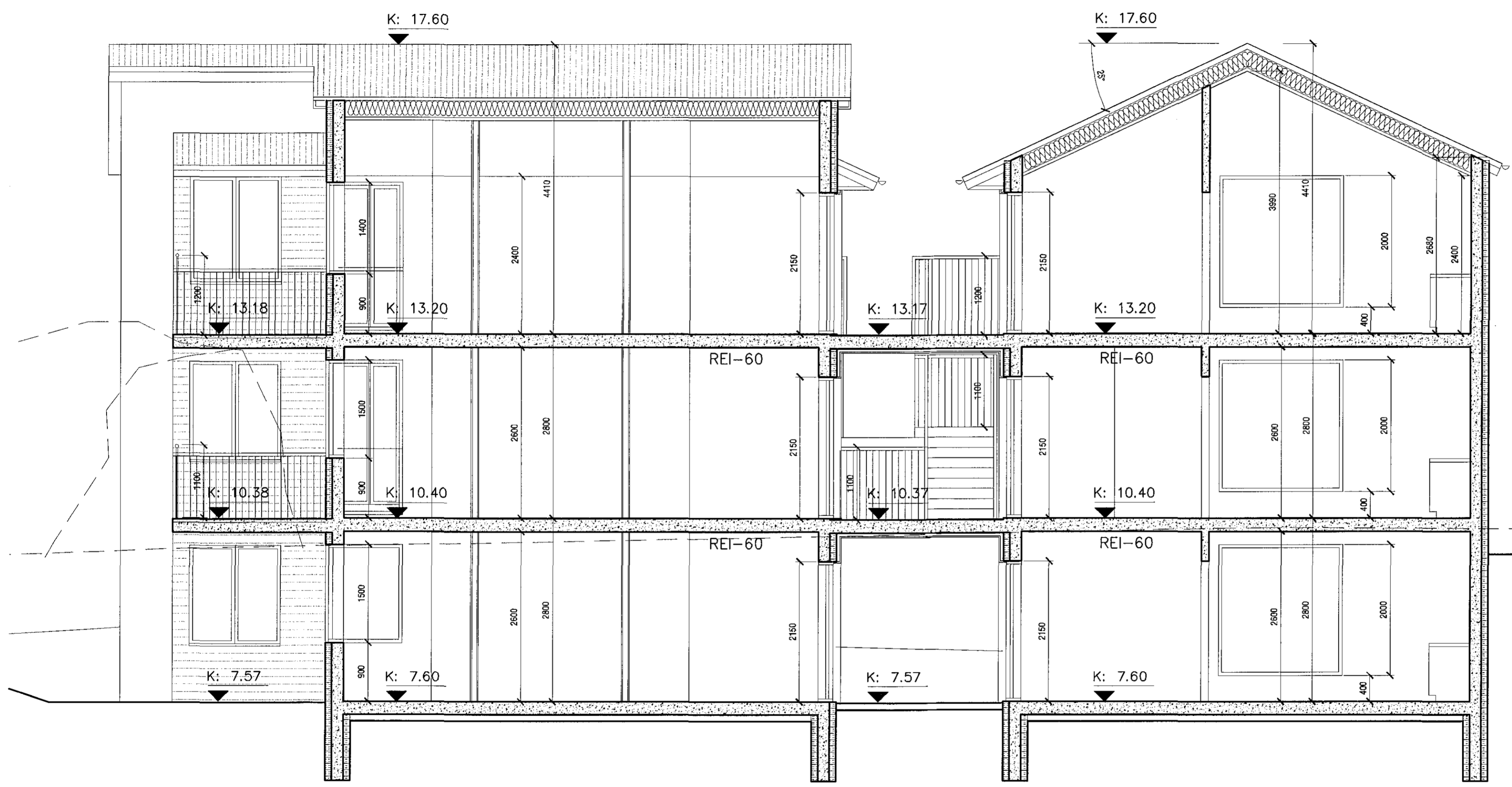
Sneiðing B-B mkv. 1:50
