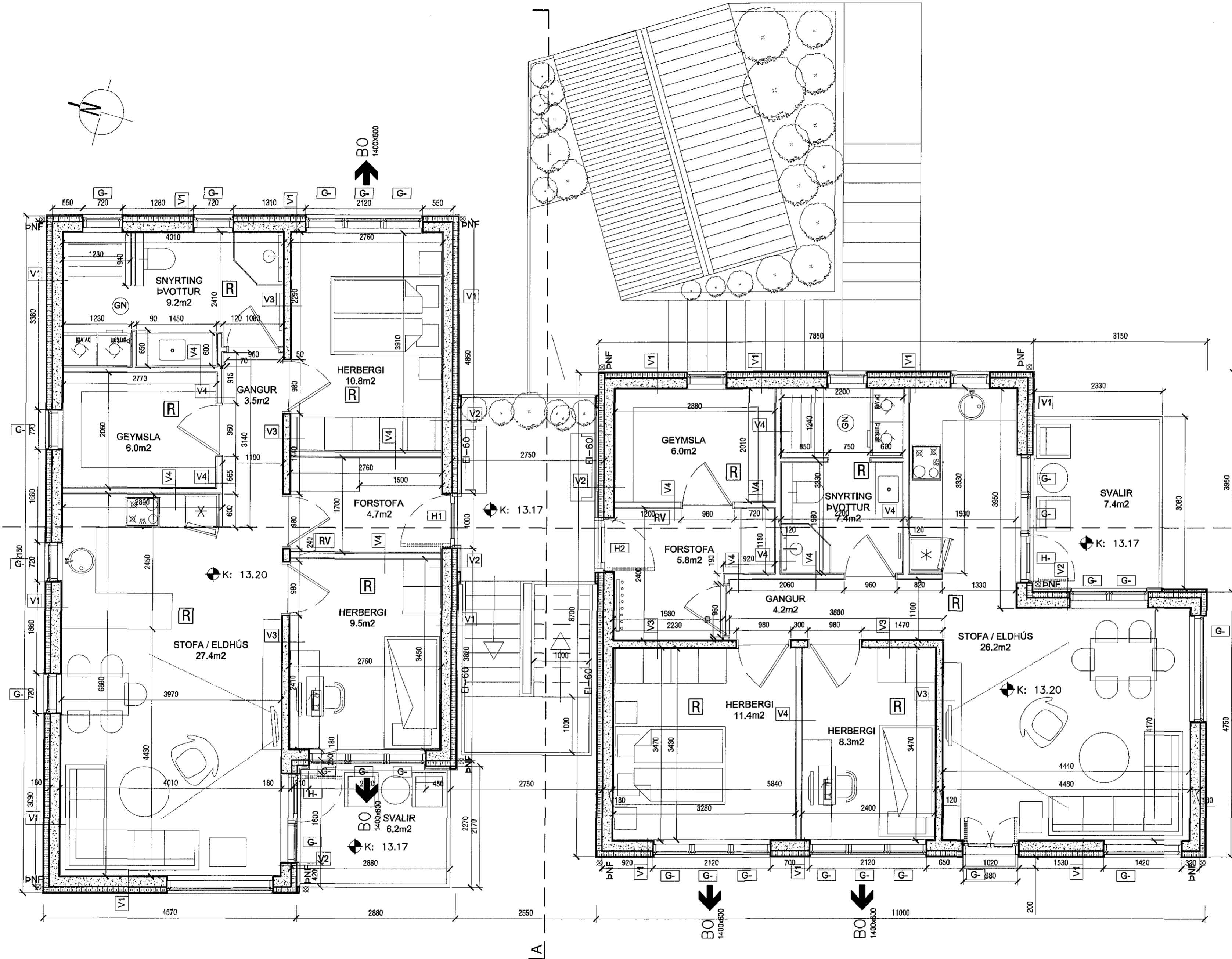
Grunnmynd - 3.hæð mkv. 1:50
