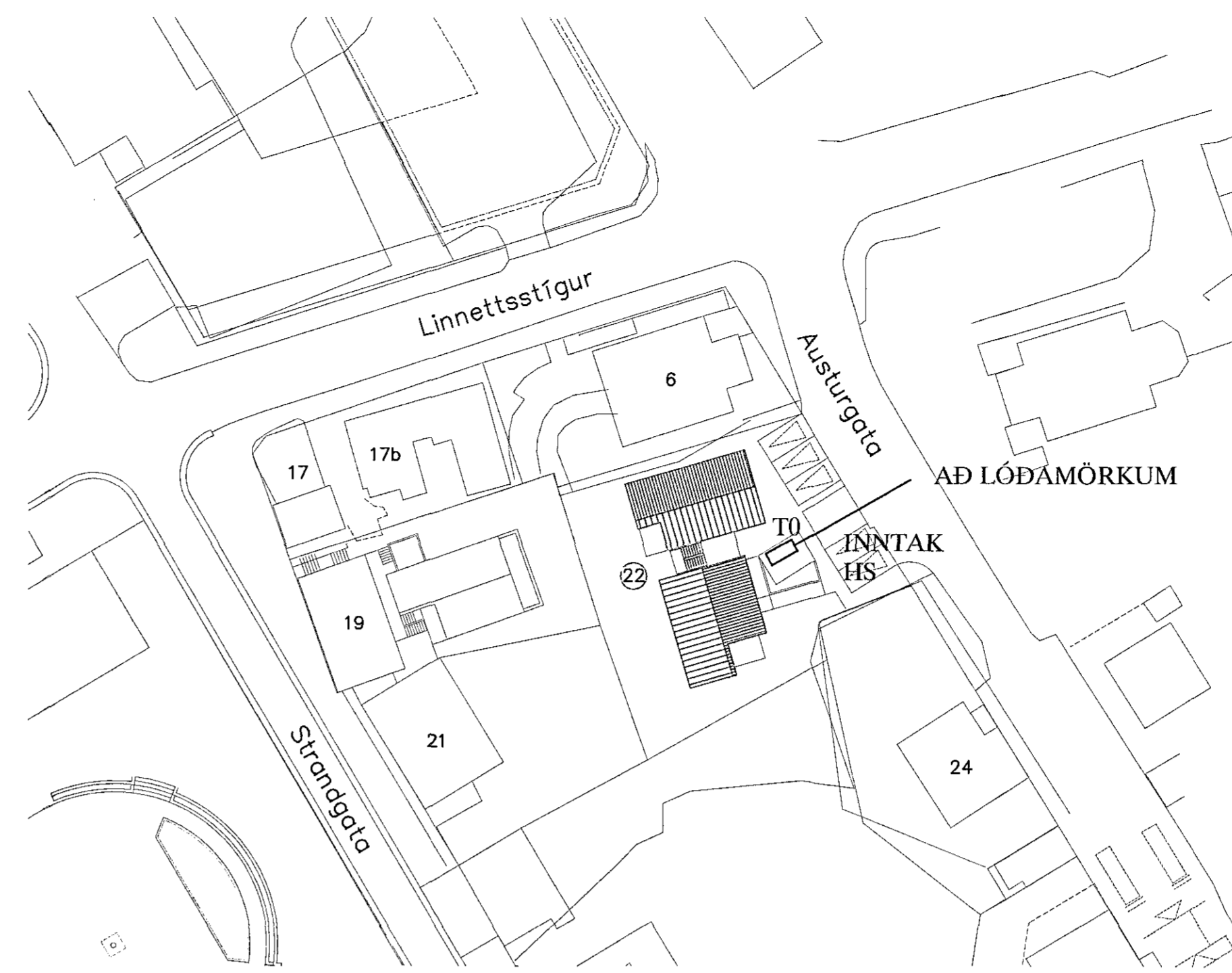
AFSTÖÐUMYND M. 1:500
