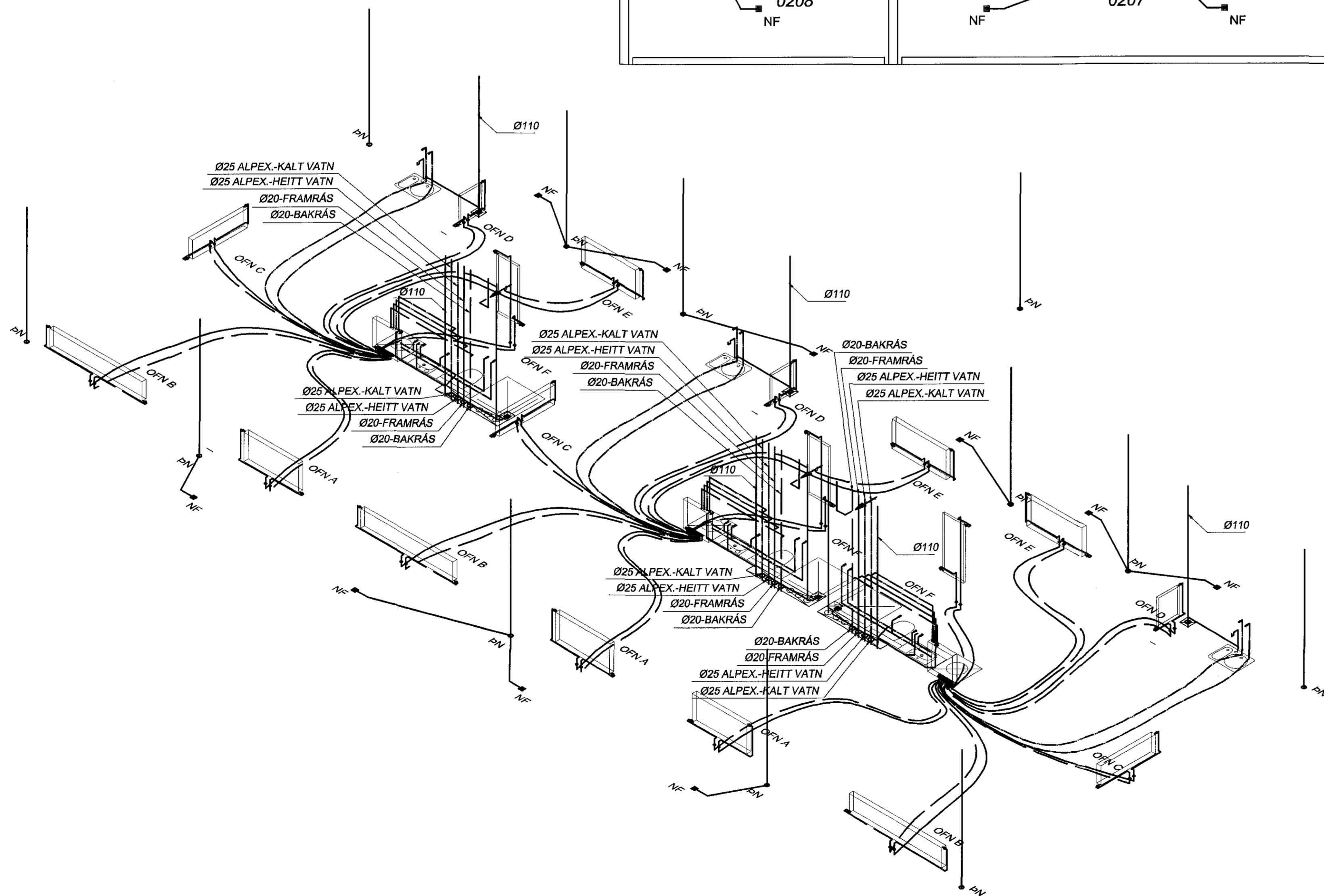
2. HÆÐ LAGNIR - RÚMMYND, 1:50
