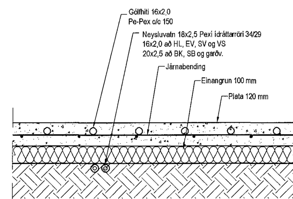
Hita- og vatnslagnir, Snið í botnplötu bilageymslu, 1:10
