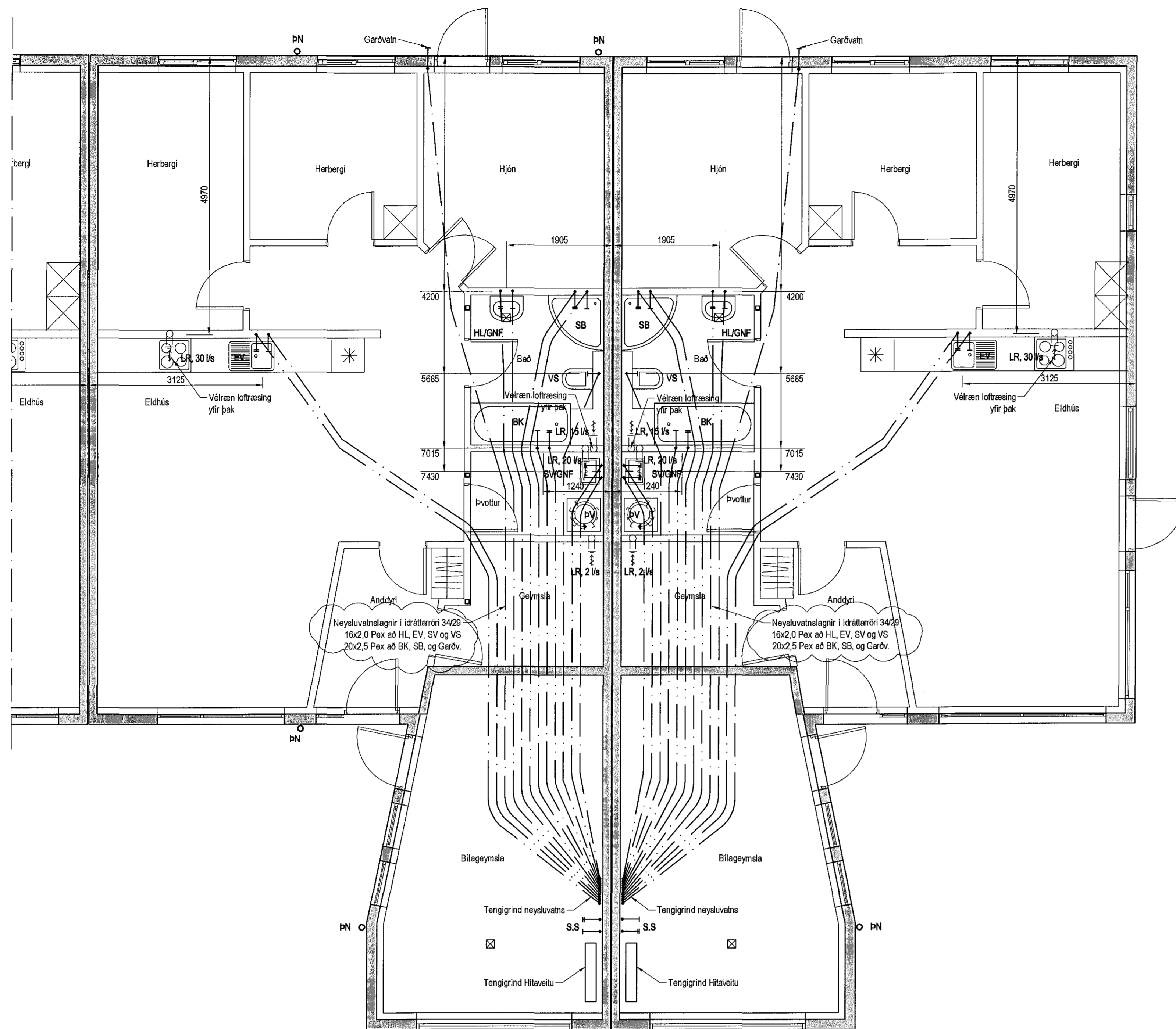
Neysluvatnslagnir 1. hæð, 1:50
