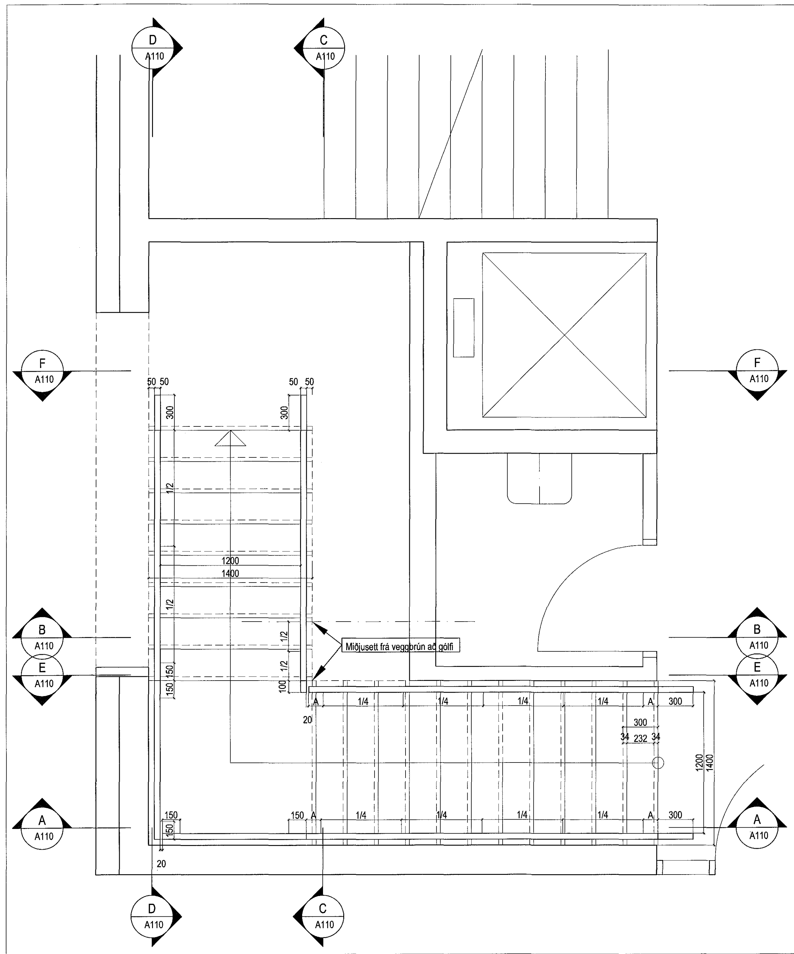
Grunnmynd 3. hæð
