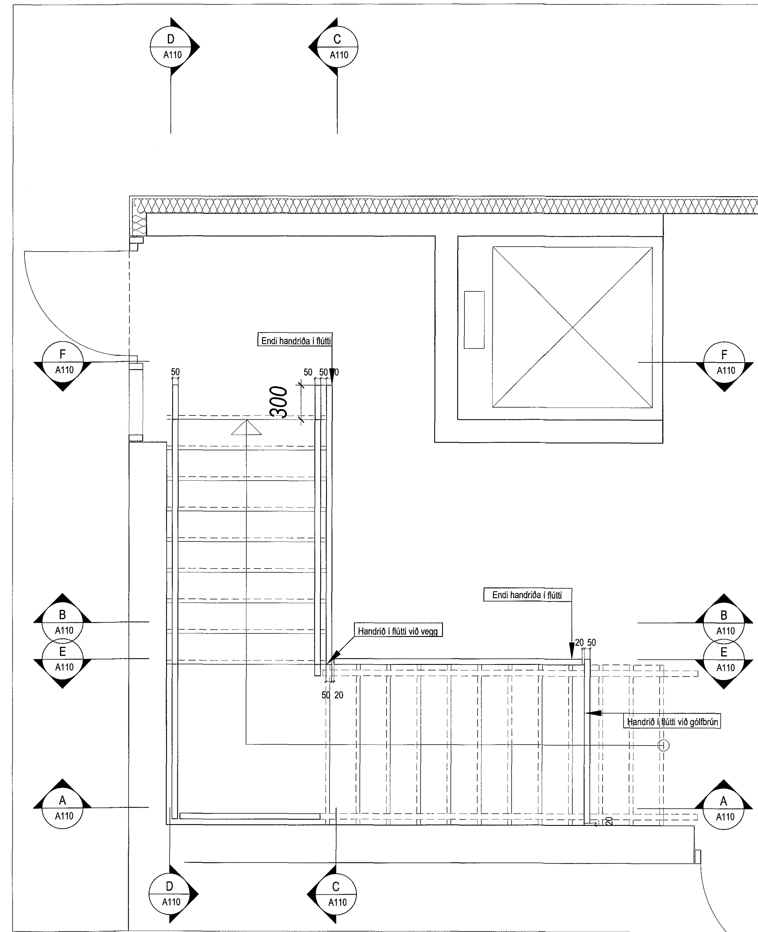
Grunnmynd 4. hæð
