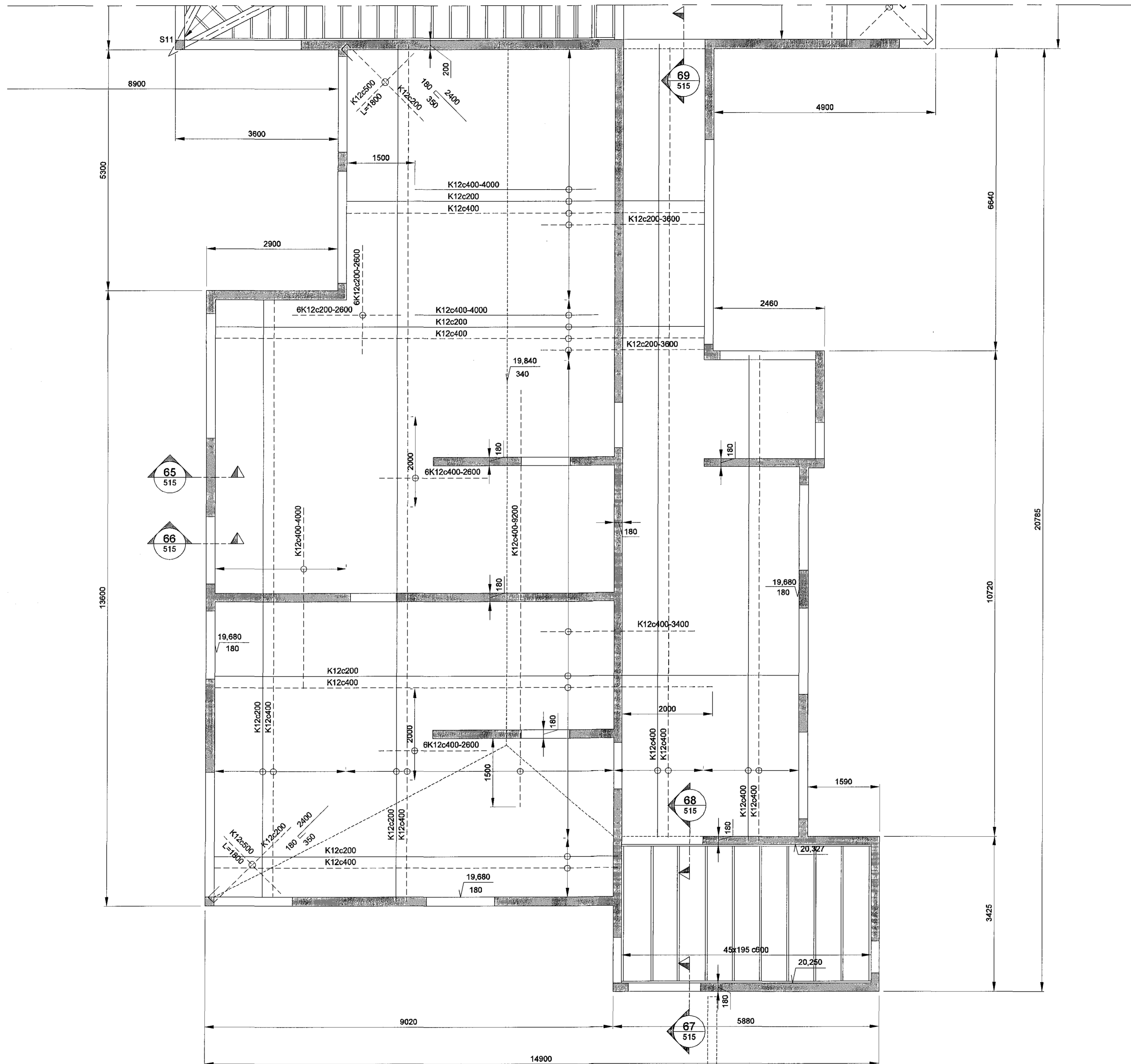
GRUNNMYND - ÞAKVIRKI MKV. 1:50 (A1)
