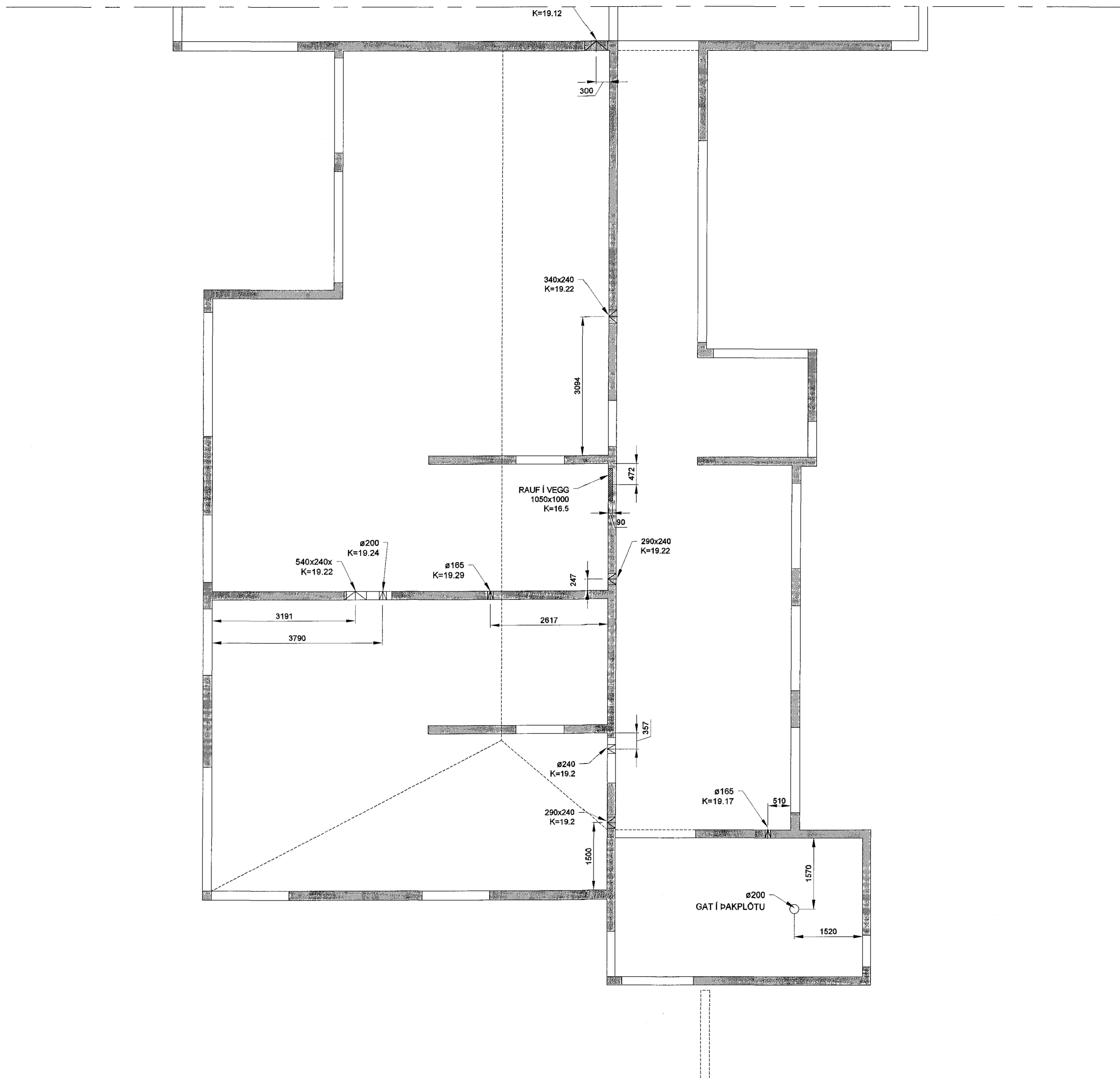
GRUNNMYND - GATAPLAN MKV. 1:50 (A1)
