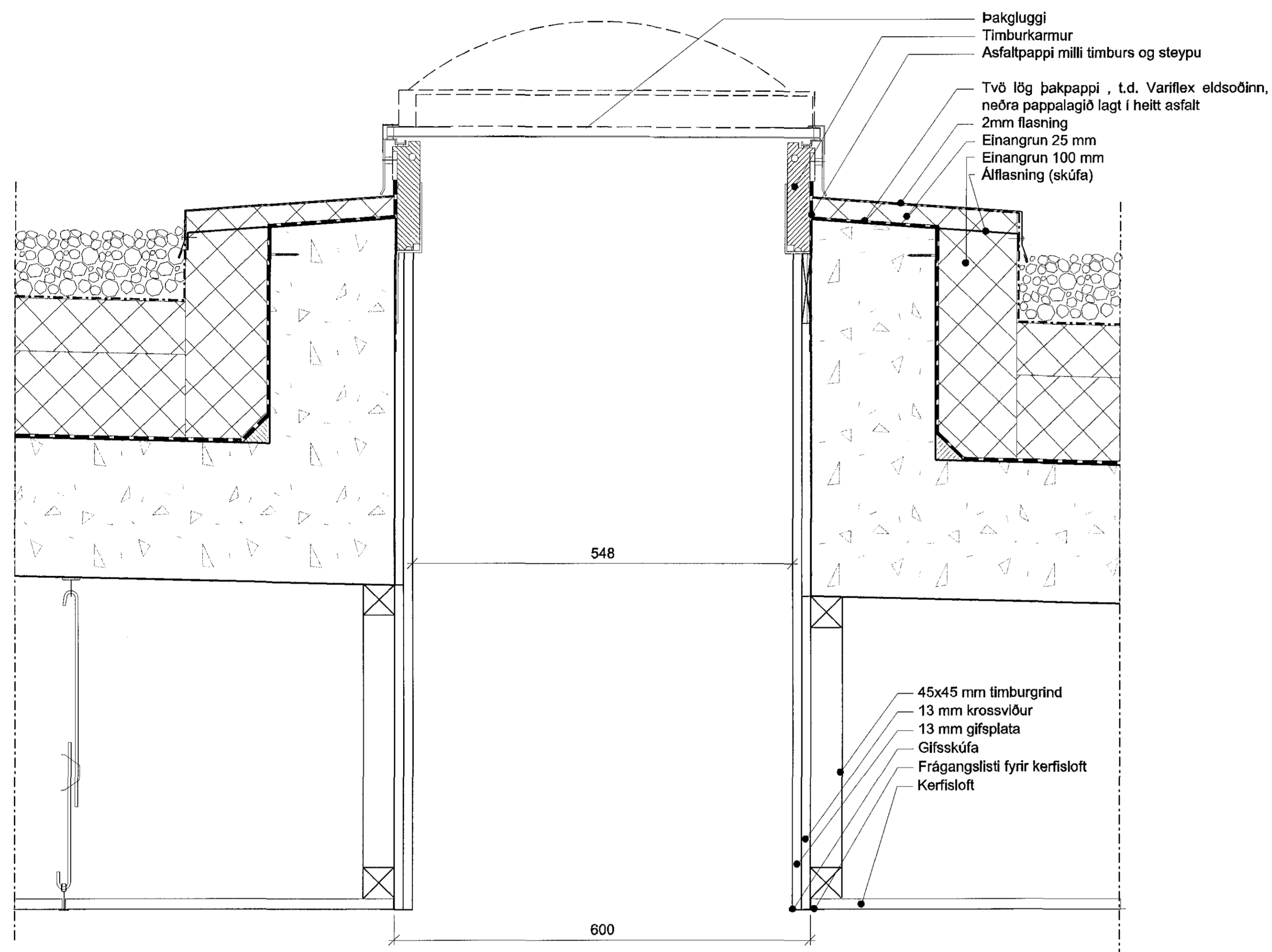
1 Lóðrétt snið - þakgluggi 39-06 1:5
