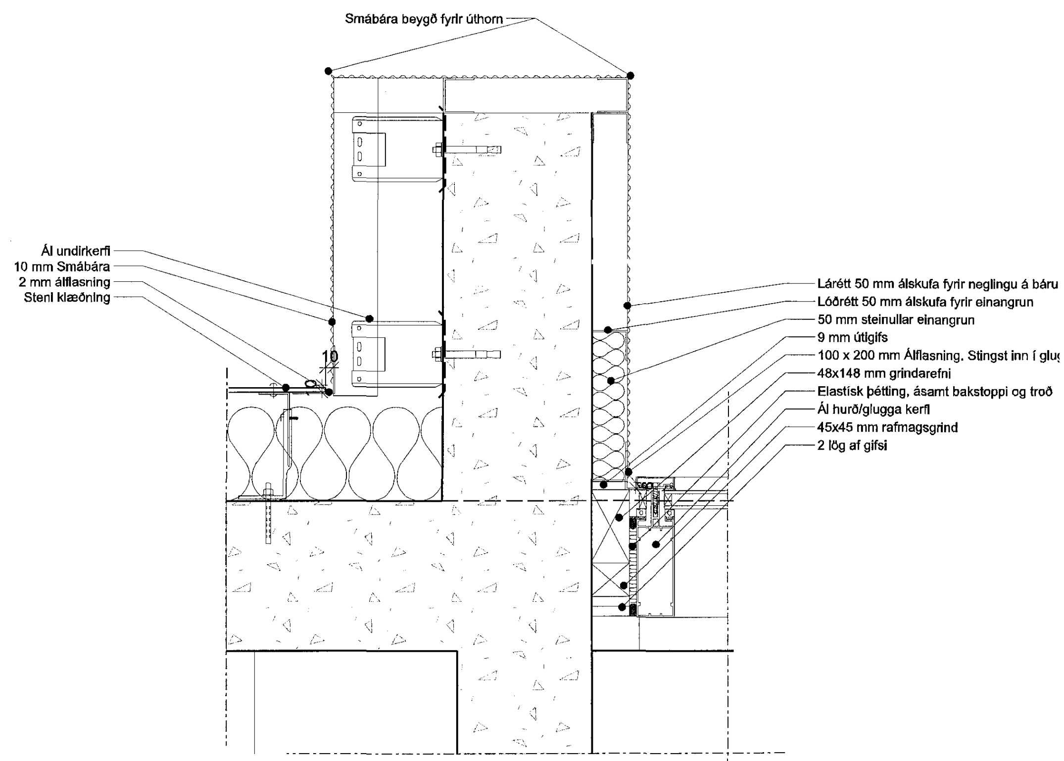
1 Lárétt deili - aðal inngangur 39-04 1:5
