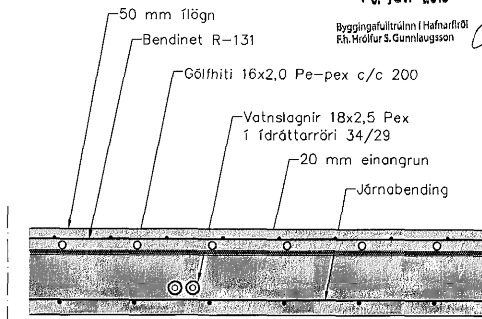
Hita- og vatnslagnir. Snið í milliplötu. 1:10
