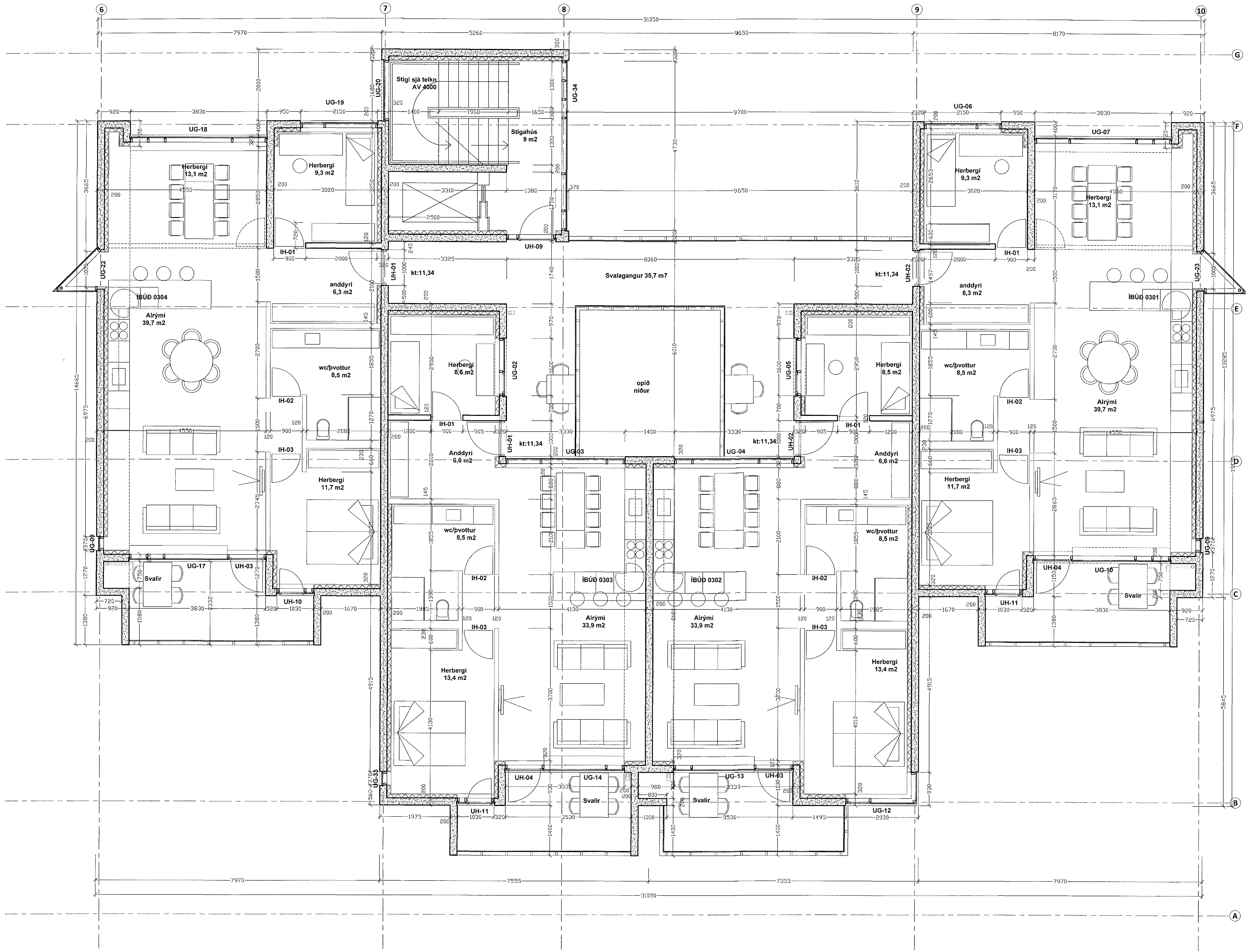
GRUNNMYND 3.HÆÐ. Mkv 1:50
