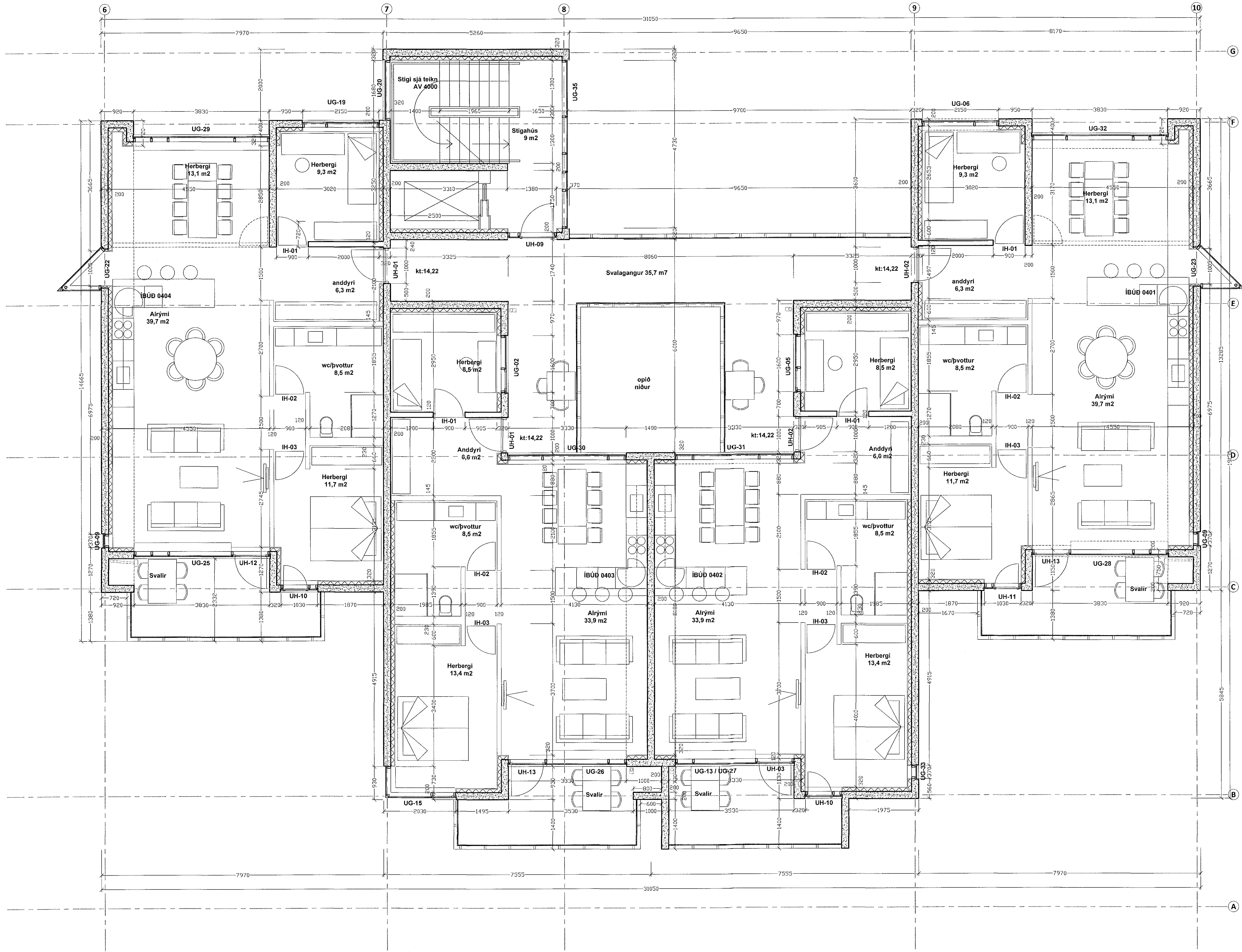
GRUNNMYND 4.HÆÐ. Mkv 1:50
