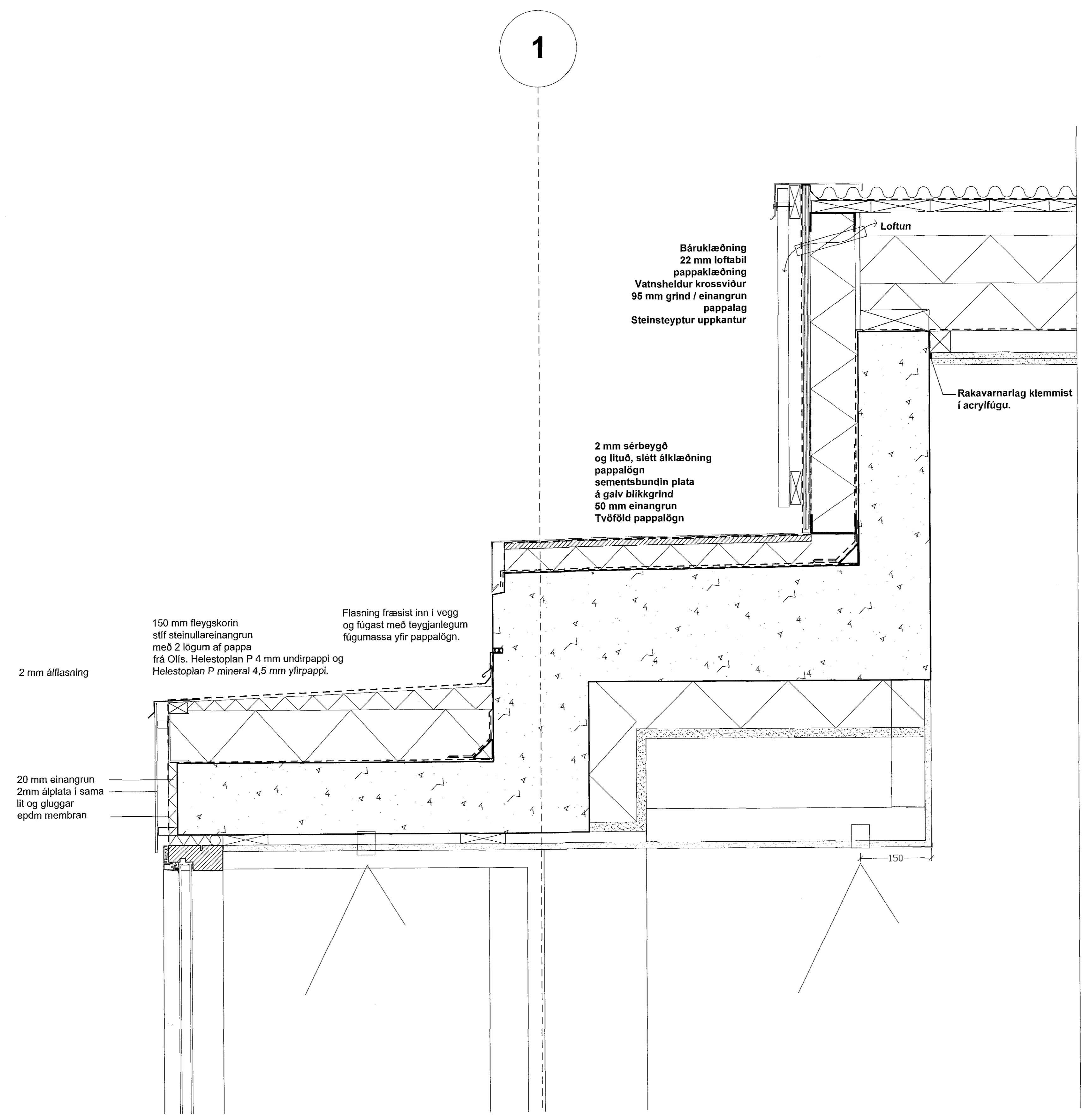
D.22 Lóðrétt sneiðing mkv 1:5
