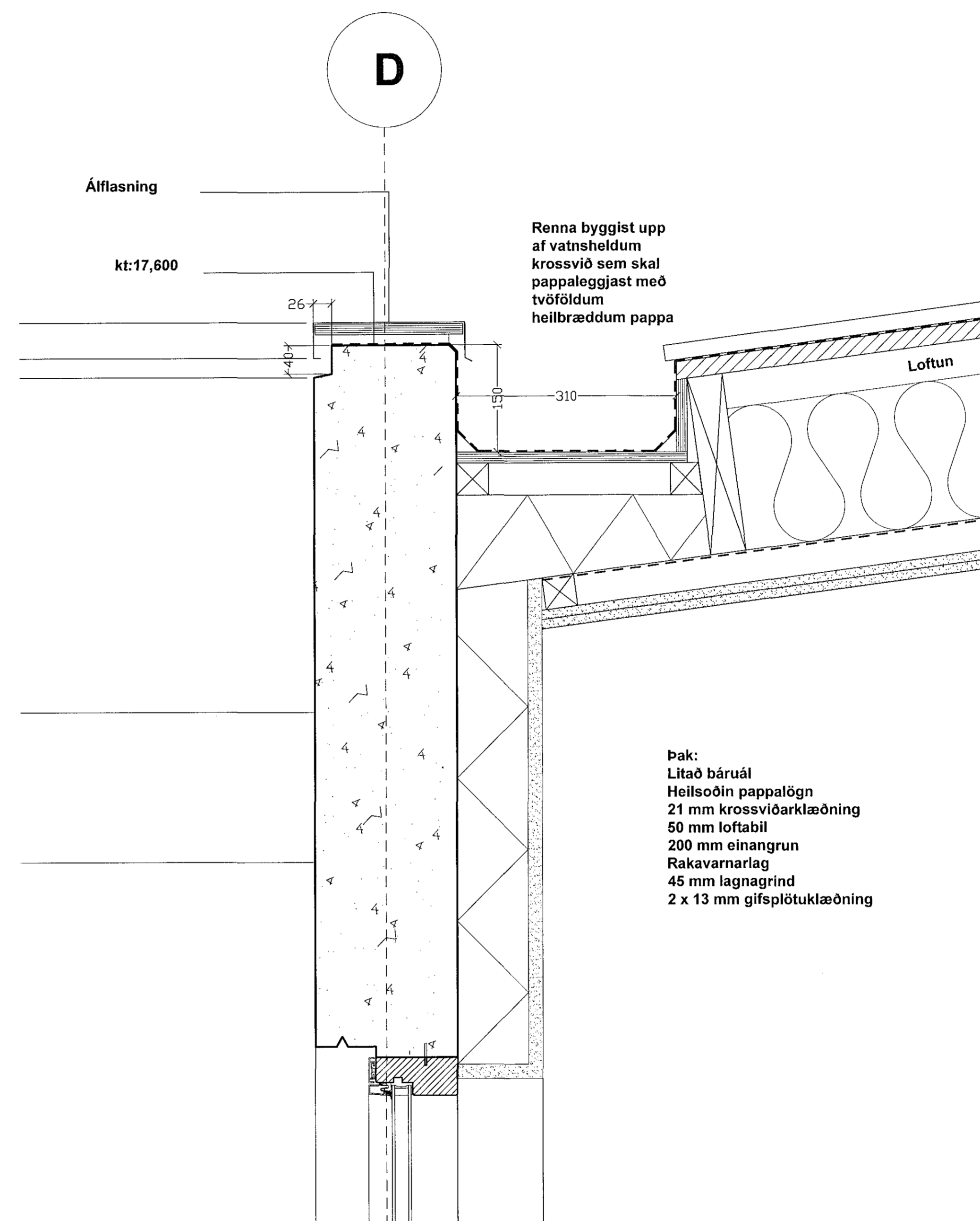
D.10 Lóðrétt sneiðing mkv 1:5
