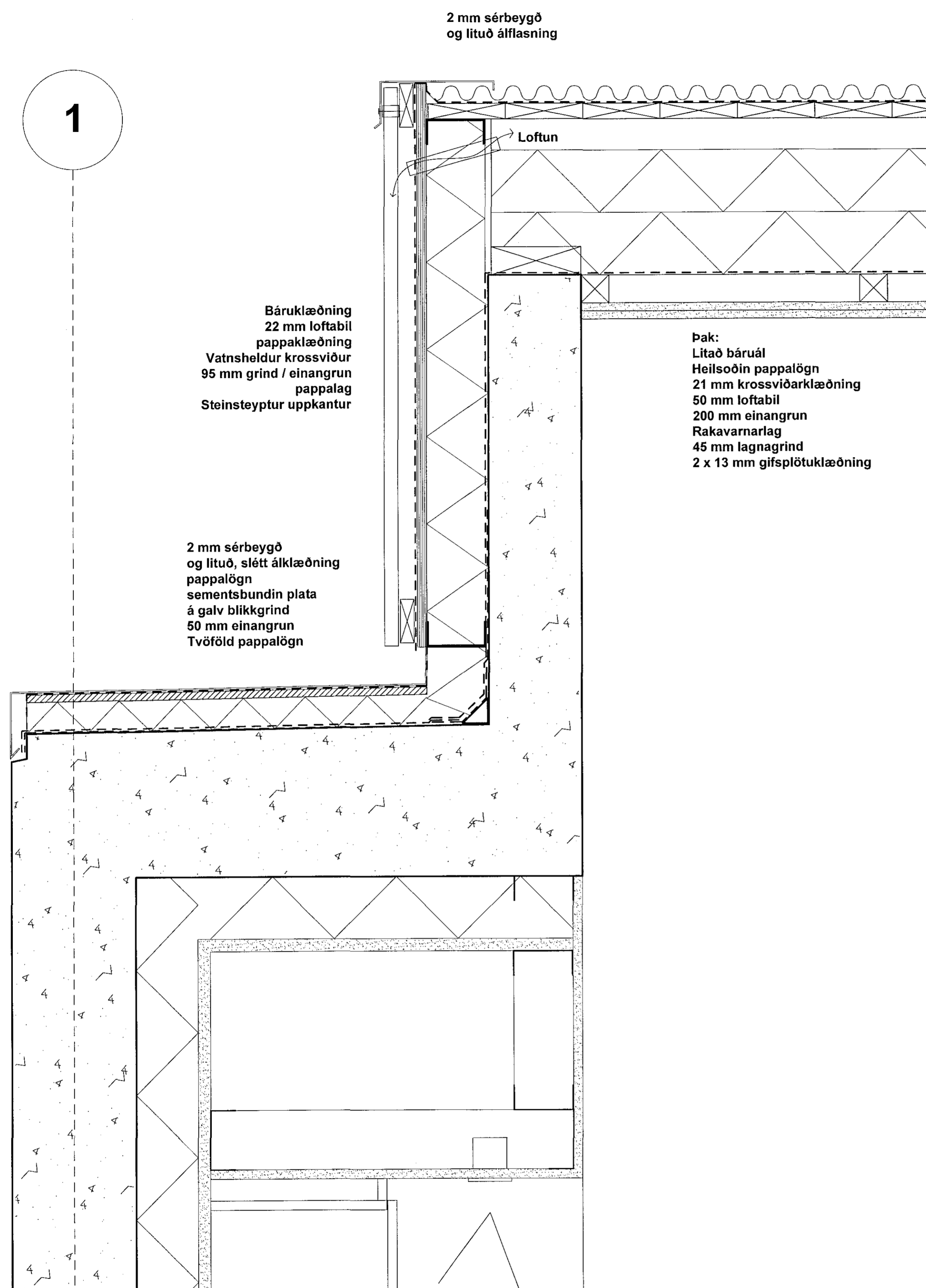
D.11 Lóðrétt sneiðing mkv 1:5
